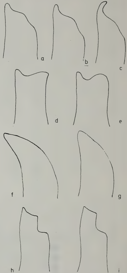
Abb. 23. Distales Ende des linken id -Seitenteils, von oben, der palaearktischen Arten von Tipula ( T. ) (a—i wie Abb. 18).
