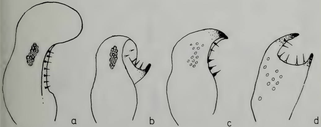
Abb. 19. id -Hinterteil, von der Innenseite, einiger afrotropischen Arten von Tipula ( T. ); a, bicolor ; b, speiseriana ; c, lobeliae ; d, capnioneura .
