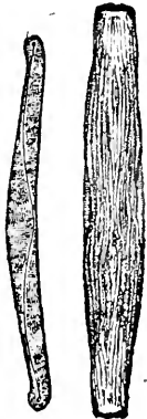
Fig. 25.— A. ( Okekenia ) inflexa .
