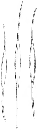
Fig. 126.— Nitzschia longissima ( Nitzschella .) var. Closterium .
