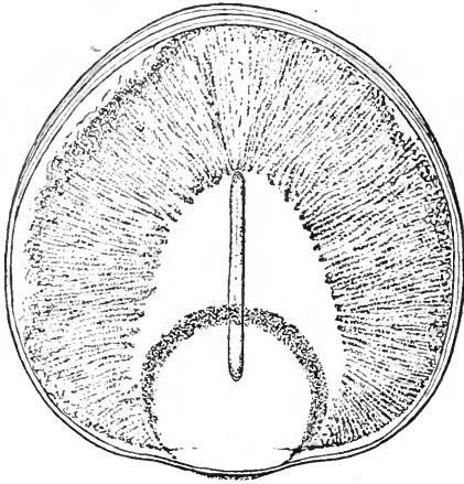
Fig. 288.— Van Heurckielia admirabilis .
