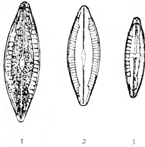
Fig. 28.—(1 2) M. lanceolata Thl.; (3) M. Smithii Thw., var. lacustris Grun.
