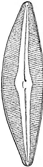
Fig. 26.— Cymbella Ehrenbergii Kütz.
