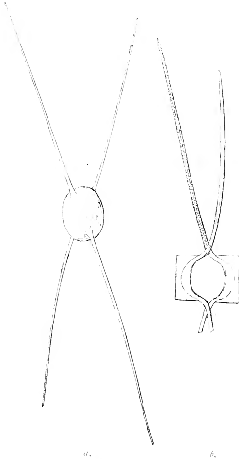
Fig. 139.— a. Chetoceros Wighamii. b. Chetoceros Lorenzianus.
