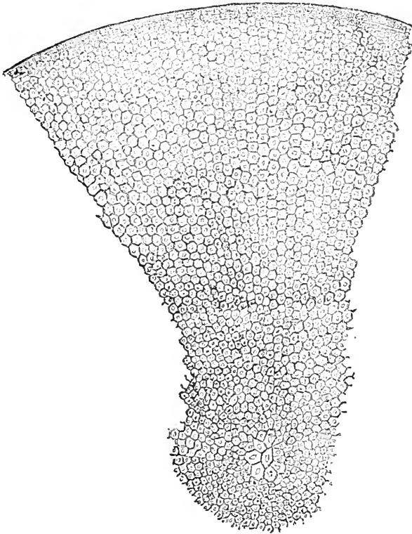
Fig. 277.— Coscinodiscus Asteromphalus var. constitua .
