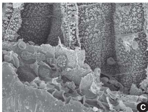
Fig. 62. Diphyscium foliosum . A – общий вид перистомы, \times 61 ; B – поверхность складчатого конуса (гомологичного эндостому) в средней его части, \times 480 ; C – основание складчатого конуса, кнаружи от которого располагается низкая мембрана, гомологичная экзостому (представлена не во всех коробочках, ср. с рис. A), \times 400 .
