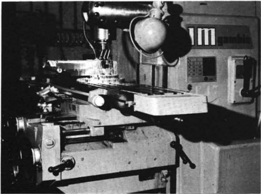
Fraiseuse GAMBIN 1M équipée de lecteurs optiques micrométriques pour les mouvements longitudinaux et transversaux.
