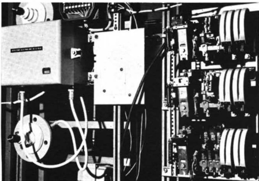
Maquette de câblage d'une installation de pompage avec détection électronique des niveaux d'eau.
