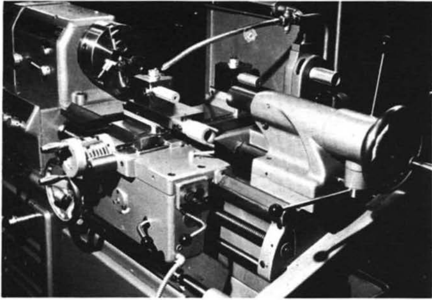
Tour RAMO POLYBUT et MICROBUT
