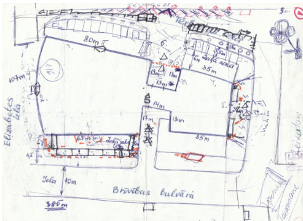
Ministru padomes ārējās aizsardzības loka barikāžu shēma. 1991. gada janvārī zīmēts oriģināls. 1991. gada barikāžu muzeja krājums.
