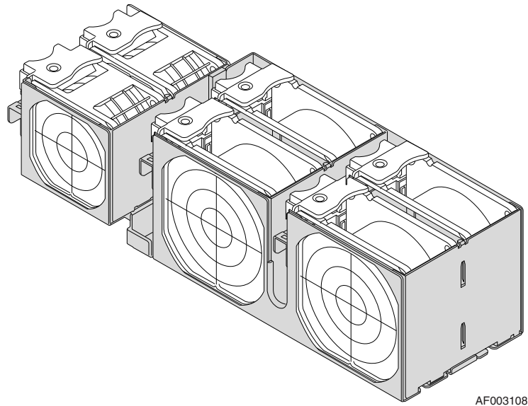
Figure 16. Fan Module Assembly
