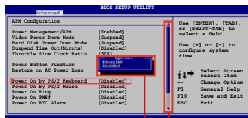
设置窗口 滚动条
