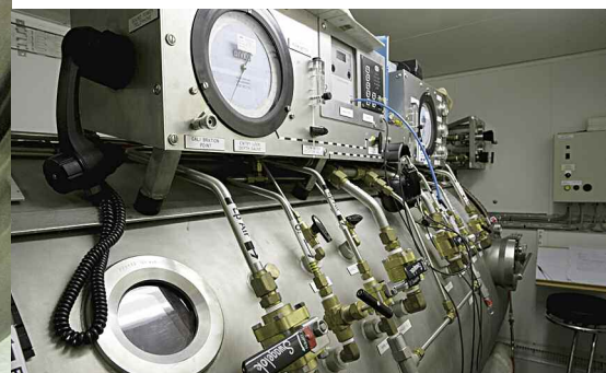
Vadības panelis ļauj precīzi mainīt gaisa spiedienu barokameras iekšienē, imitējot cilvēka atrašanos dažādā dziļumā.
