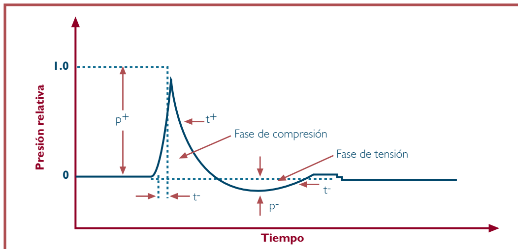
Figura 1. Diagrama ideal de la onda de choque.
