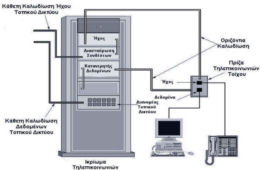
Εικόνα 10.2: Τυπικά στοιχεία που υπάρχουν στην οριζόντια καλωδίωση ενός ορόφου. (Τροποποιημένη από πηγή: Oliviero, A., & Woodward, B., Cabling - The Complete Guide to Network Wiring )
