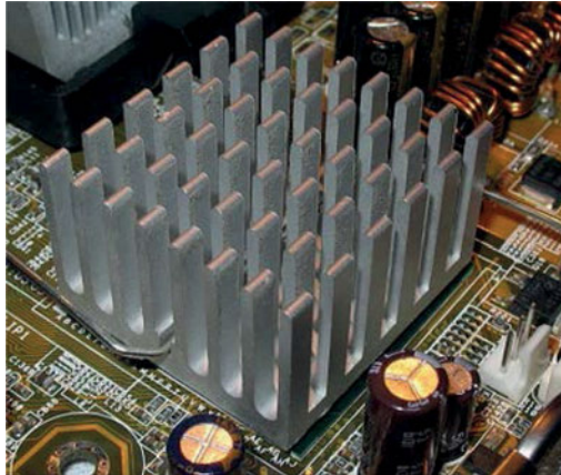
Εικόνα 2.2: Ψύκτρα
