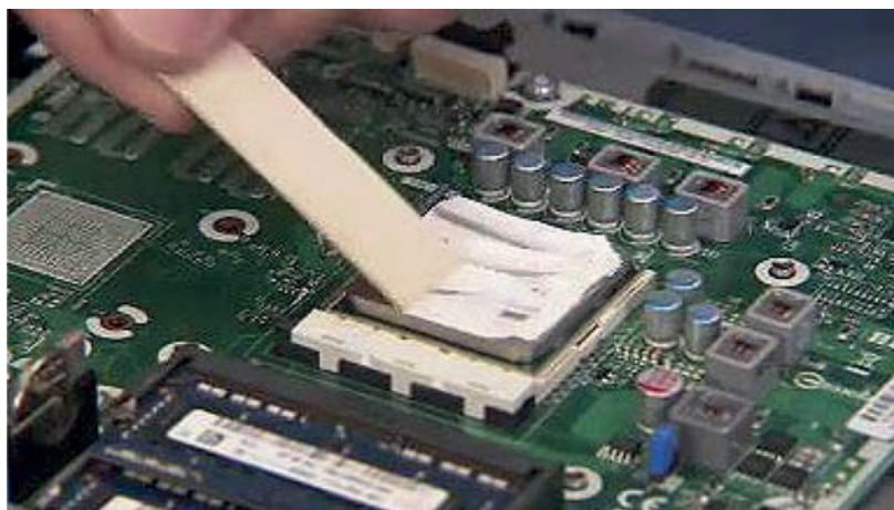
Εικόνα 2.7: Εφαρμογή θερμοαγώγιμης πάστας
