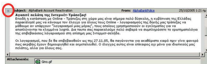
Εικόνα 8.4: Παραπλανητικό e-mail
