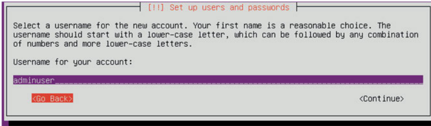
Εικόνα 7.19: Δημιουργία χρήστη
