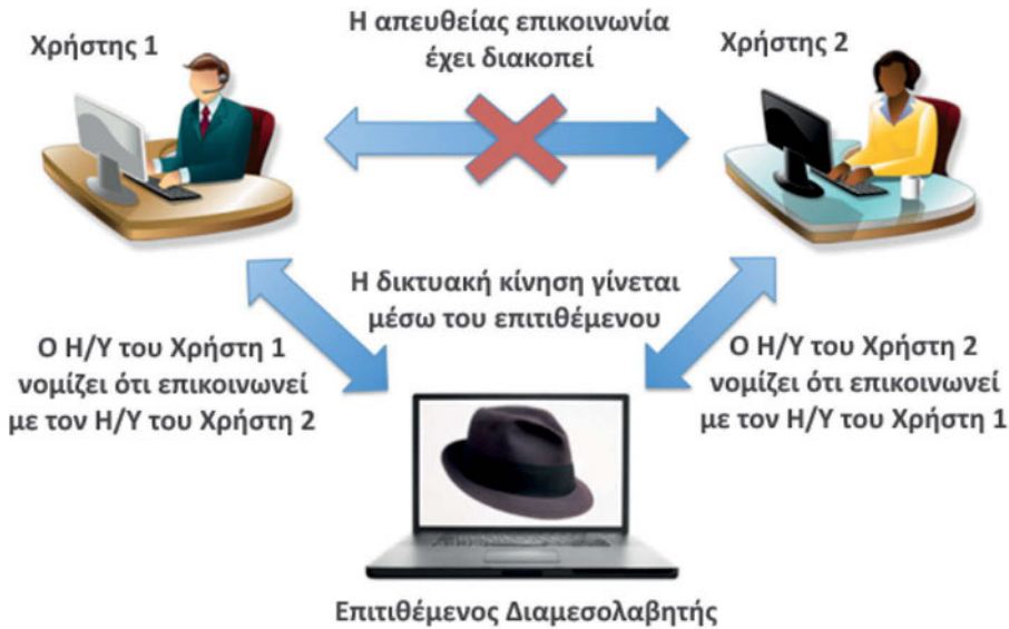
Εικόνα 8.1: Επίθεση Διαμεσολαβητή
