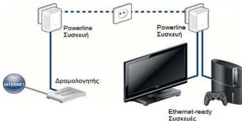
Εικόνα 11.1: Τρόπος εγκατάστασης της τεχνολογίας Powerline σε ένα σπίτι ή μικρό γραφείο
