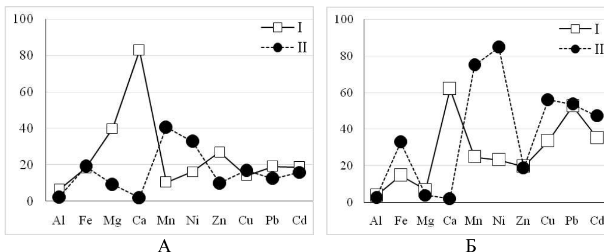
Рис. 2. Для подвижных форм химических элементов, извлекаемых раствором серной кислоты (I) и раствором Тамма (II), от их валового содержания в конкрециях, выделенных из образцов криометморфических горизонтов CRM2g, глубина 70–95 см (А) и CRM3g, глубина 125–142 см (Б)
