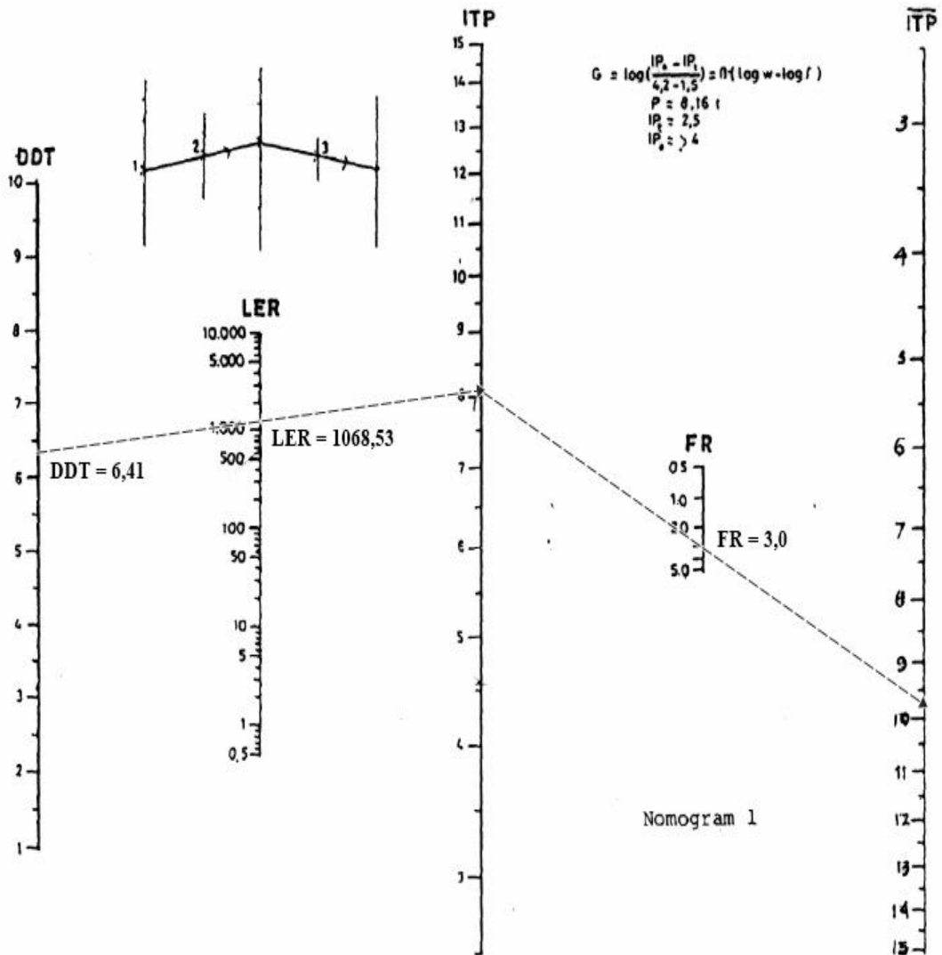
Gambar 4.12 Nilai ITP Berdasarkan Nomogram 1
