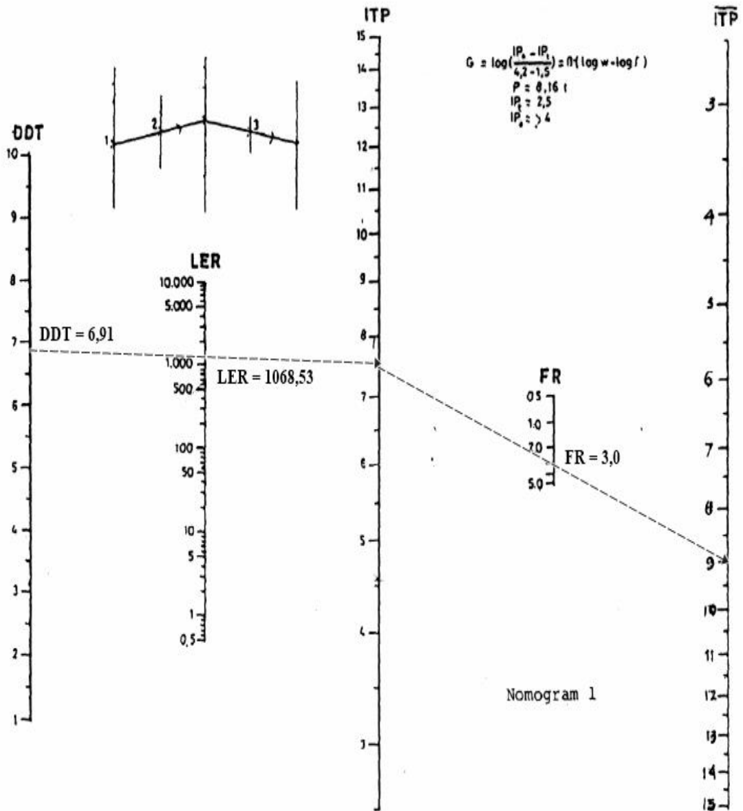
Gambar 4.10 Nilai ITP Berdasarkan Nomogram 1
