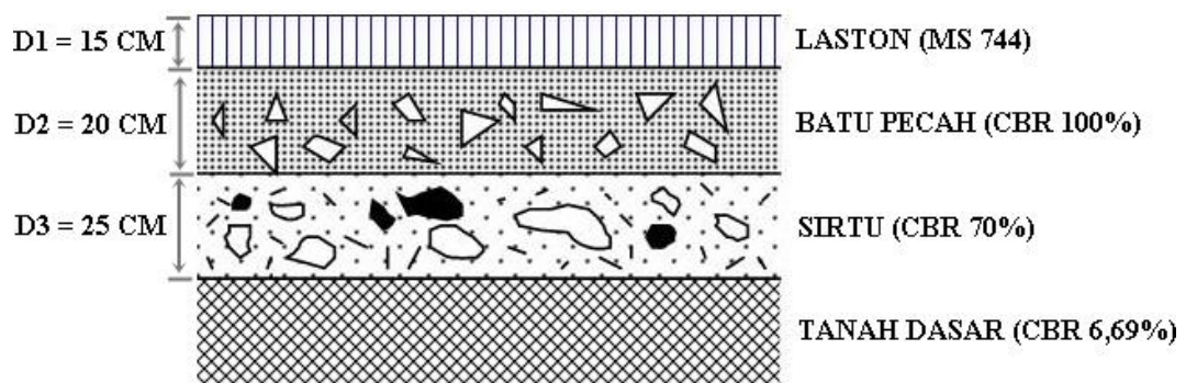
Gambar 4.22 Susunan Perkerasan Segmen 9
