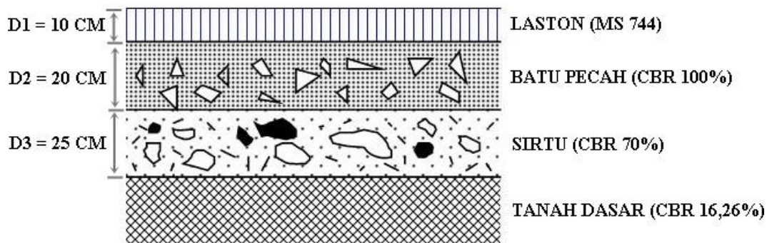
Gambar 4.19 Susunan Perkerasan Segmen 6
