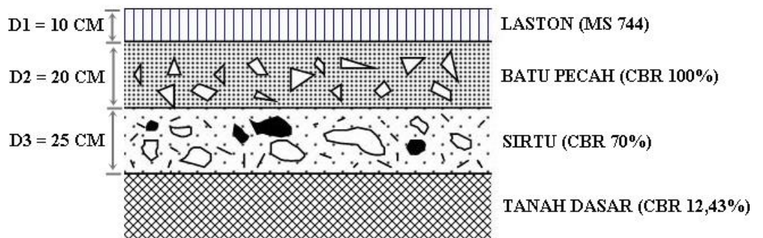
Gambar 4.21 Susunan Perkerasan Segmen 8
