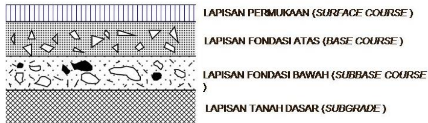
Gambar 2.2 Susunan Lapisan Perkerasan
