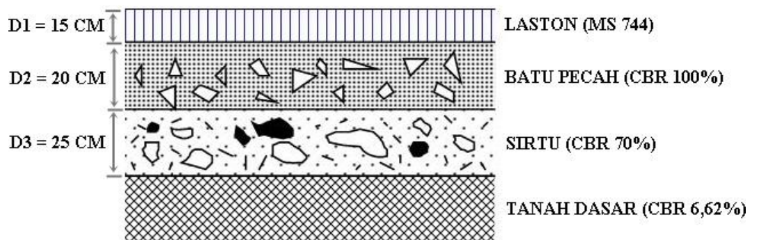
Gambar 4.18 Susunan Perkerasan Segmen 5
