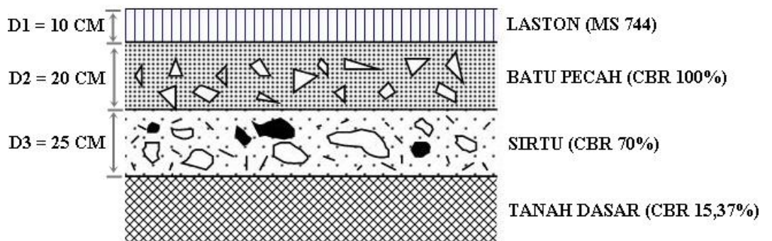
Gambar 4.15 Susunan Perkerasan Segmen 2
