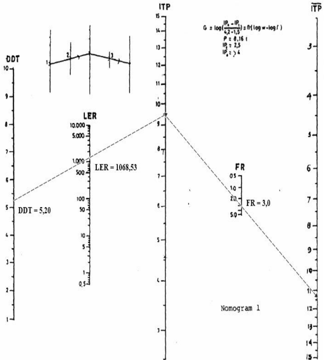
Gambar 4.11 Nilai ITP Berdasarkan Nomogram 1
