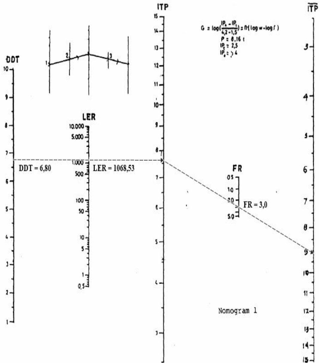
Gambar 4.6 Nilai ITP Berdasarkan Nomogram 1
