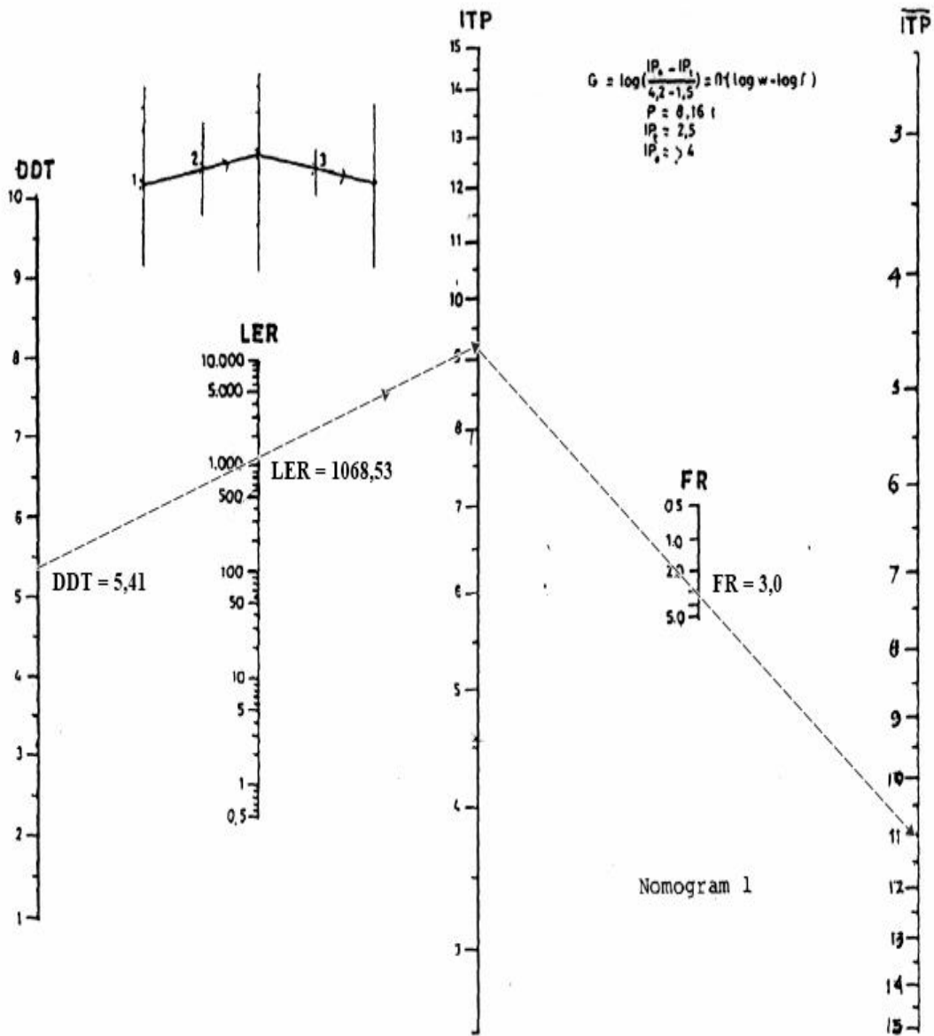
Gambar 4.5 Nilai ITP Berdasarkan Nomogram 1
