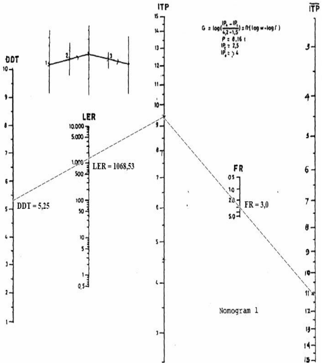
Gambar 4.13 Nilai ITP Berdasarkan Nomogram 1
