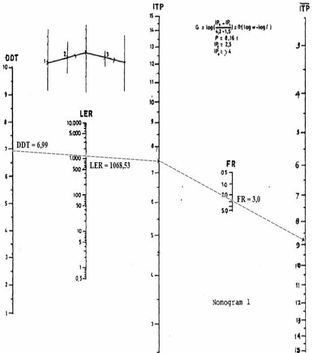
Gambar 4.8 Nilai ITP Berdasarkan Nomogram 1
