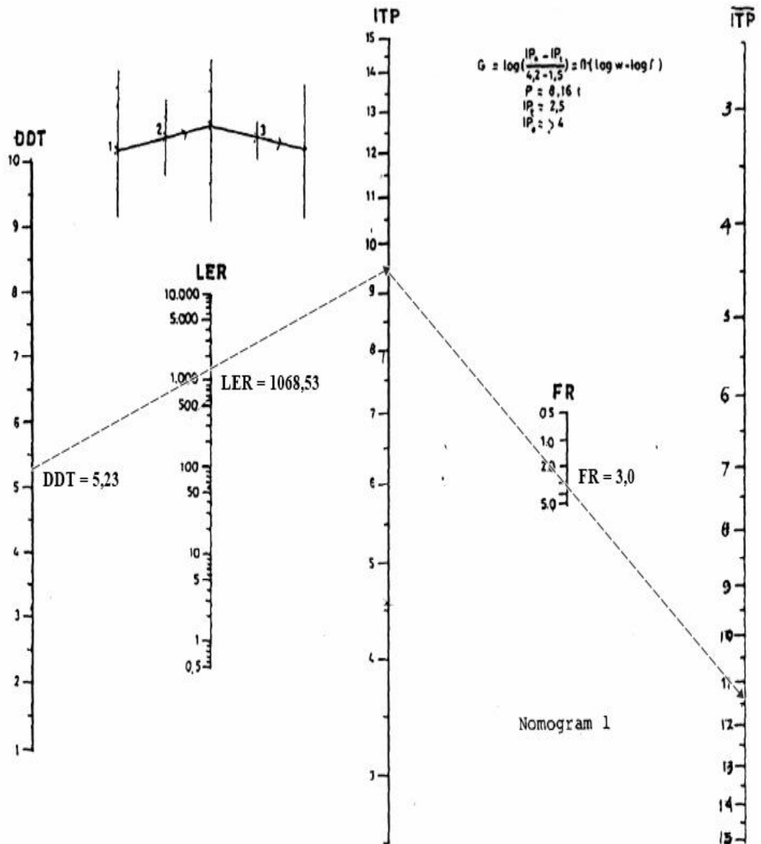
Gambar 4.9 Nilai ITP Berdasarkan Nomogram 1
