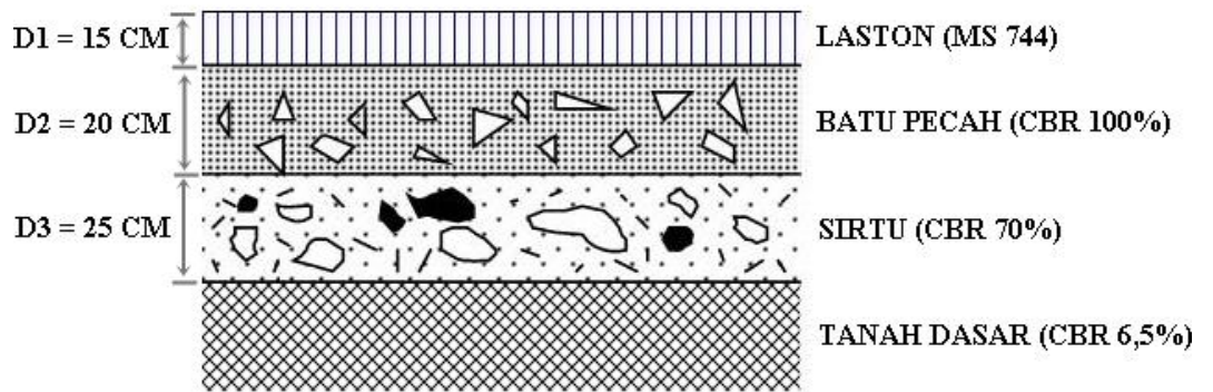
Gambar 4.20 Susunan Perkerasan Segmen 7
