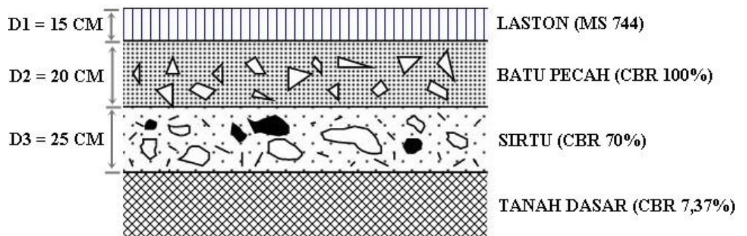
Gambar 4.16 Susunan Perkerasan Segmen 3
