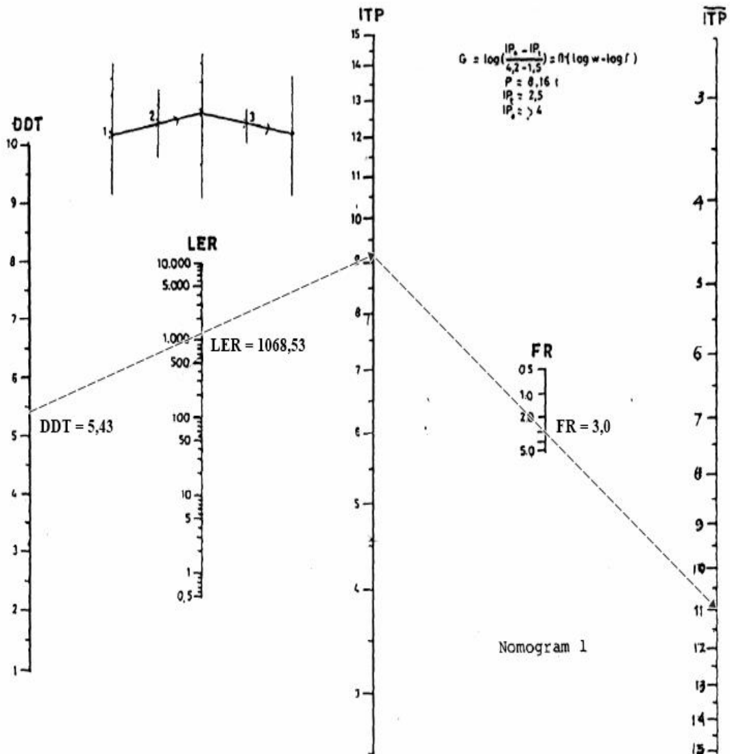
Gambar 4.7 Nilai ITP Berdasarkan Nomogram 1
