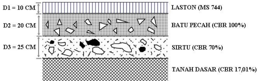
Gambar 4.17 Susunan Perkerasan Segmen 4
