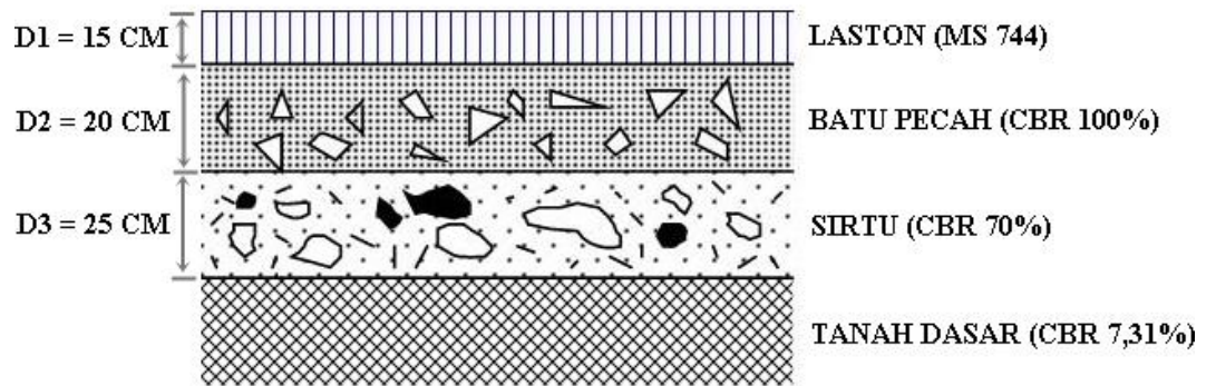
Gambar 4.14 Susunan Perkerasan Segmen 1
