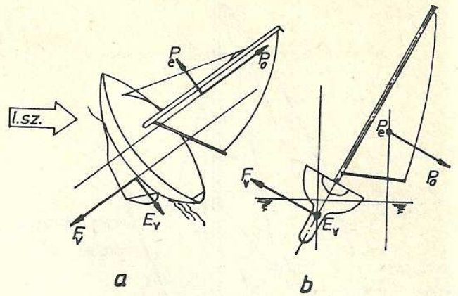
22. ábra. Az erők egyensúlya megdőlt hajó esetén a) felülnézet; b) hátnézet
