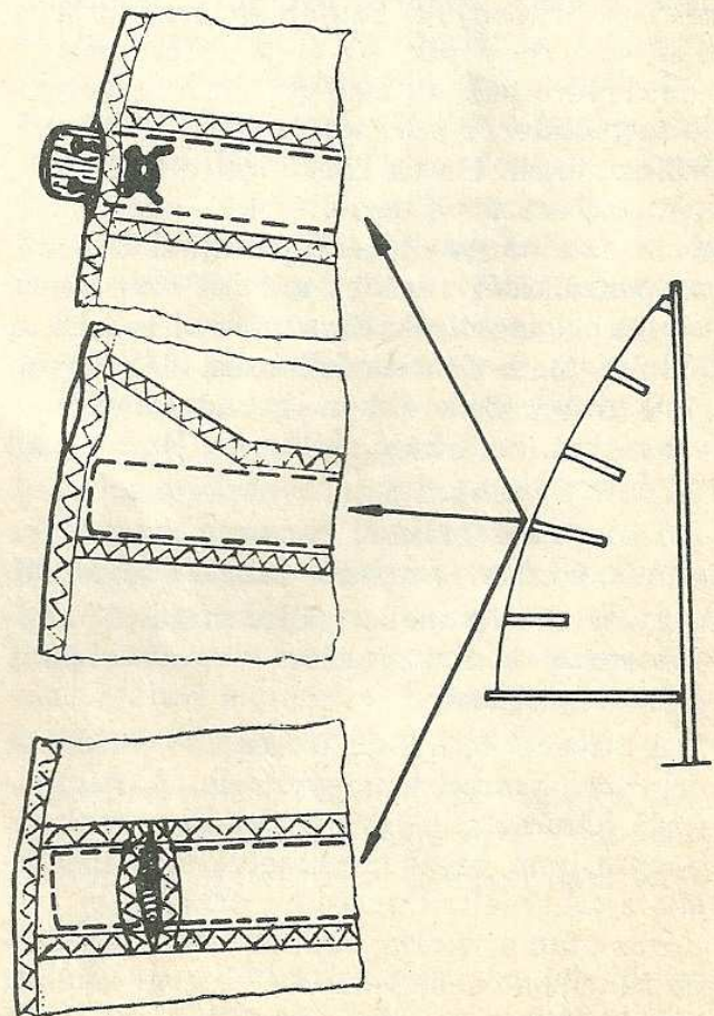
30. ábra. Vitorlaléc (lattan) rögzítése
