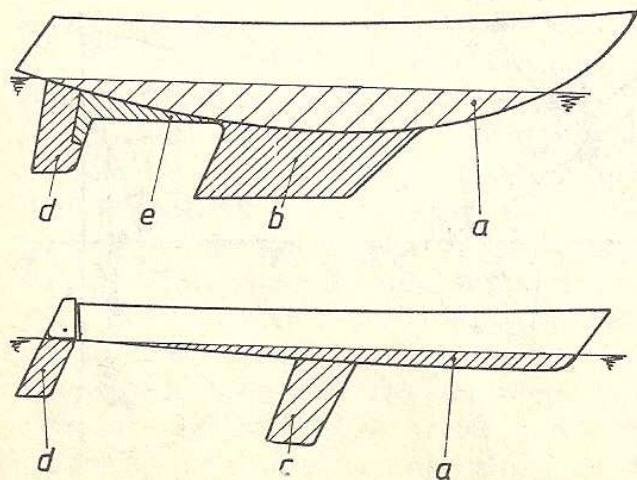
5. ábra. A laterálfelület részei
