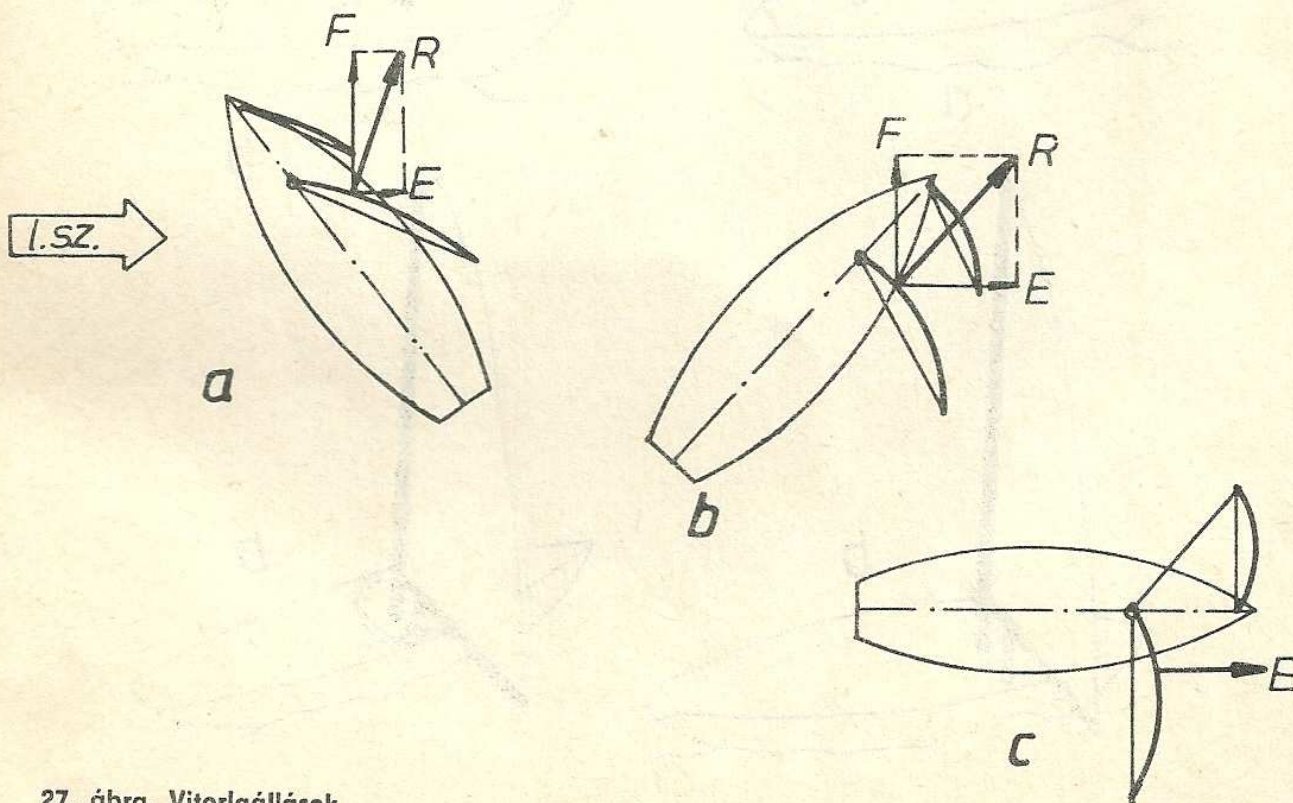
27. ábra. Vitorlaállások
