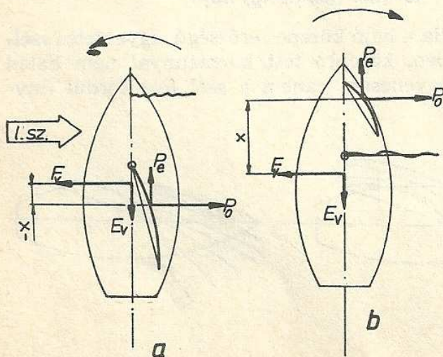
26. ábra. Kormányzás a vitorlakkal a) túlhúzott nagyvitorla, túlengedett orrvitorla: felmenetel (luvgierig hajó); b) túlhúzott orrvitorla, túlengedett nagyvitorla: leesés (leegierig hajó)
