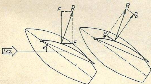
19. ábra. A vitorlán keletkező erők l.sz.: látszólagos szél; F : felhajtóerő; E : ellenállás; R : eredő; P_e : előrehajtó erő; P_o : oldalra hajtó erő
