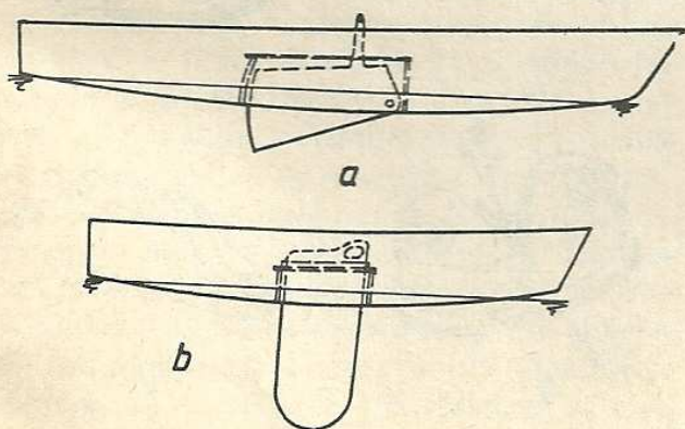
9. ábra. Uszonykialakítások a) csap körül elforgatható; b) függőle- sen leereszthető és felhúzható
