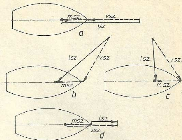
16. ábra. A látszólagos szél
