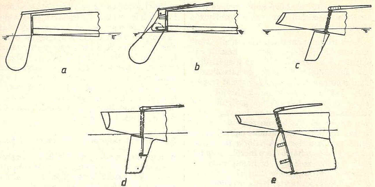
10. ábra. Kormánykialakítások
