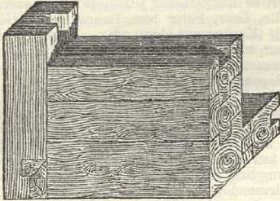
2. Ábra. Szádalt fal.
