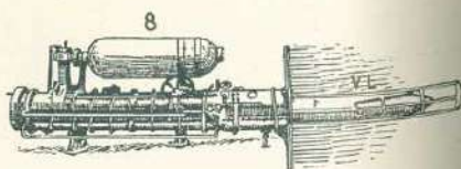
8. ábra. Vízalatti oldal-torpedócső, kilövés levegővel.
