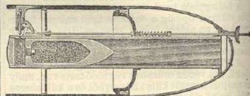
A Davis-féle lövedékes torpedó feje.
