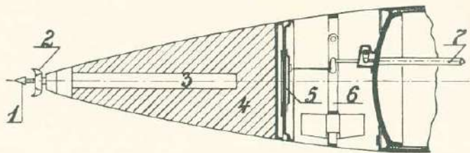
3. és 4. számú ábra. - Az 53cm-es torpedó feje és középső része a vezetőlécczel.
