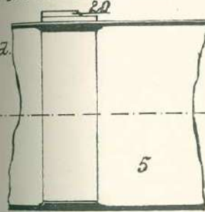
5.sz. ábra. Az 53cm-es torpedó hátsó része.
