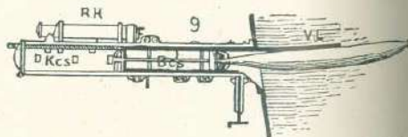
9. ábra. Vízalatti oldal-torpedócső, robbanással való kilövés közben.
