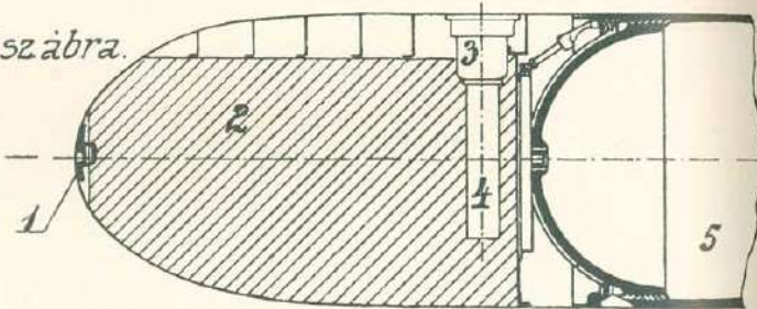
5.sz. ábra. Az 53cm-es torpedó hátsó része.
