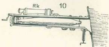
10. ábra. Vízalatti oldal-torpedócső, robbanással való kilövés előtt.
