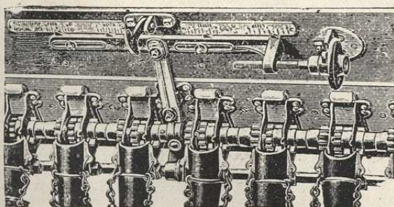
3. ábra. Tolőrendszerű magelosztók.
