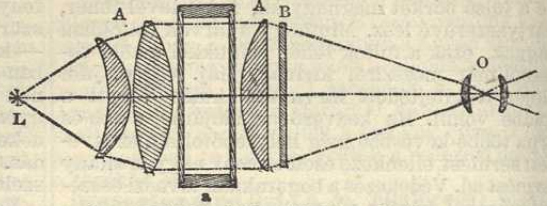
2. ábra. Vetítőkészülék optikai berendezése.
