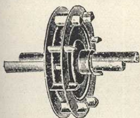
2. ábra. Merítőkanalas magelosztó.
