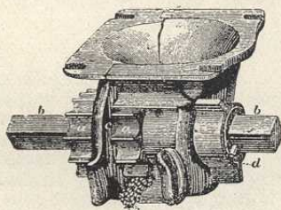
4. ábra. Hoosier-féle tolőhengeres magelosztó.
