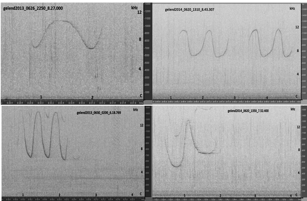
Рис. 6. Примеры спектрограмм некоторых «свистов-автографов» афалин, зарегистрированные в акватории г. Геленджик.
