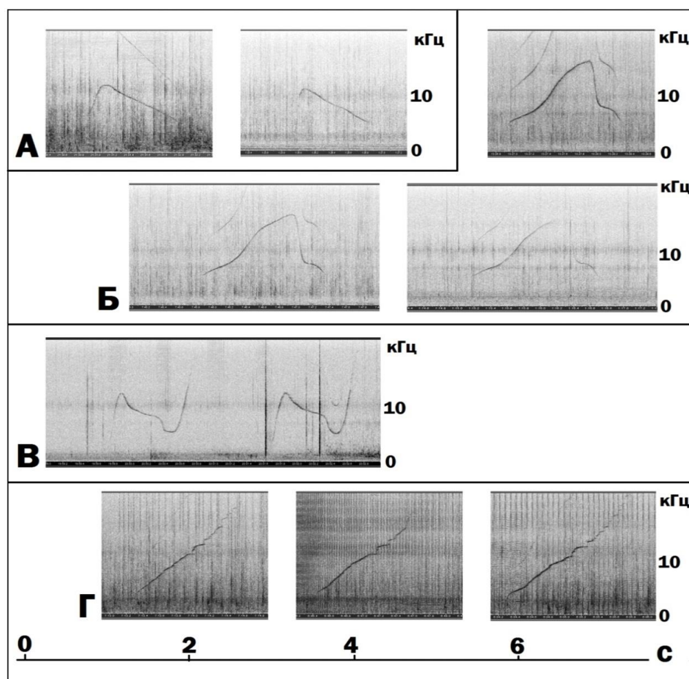
Рис. 4. Примеры спектрограмм некоторых из «свистов-автографов», зарегистрированных в акватории г. Судак – пгт. Новый Свет
