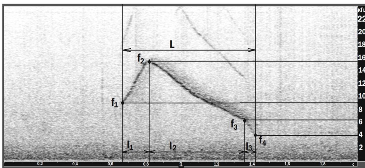
Рис. 3. Структура типичного «свиста-автографа» (по: Агафонов и др., 2016): L – общая длительность сигнала, l_1 - l_3 – длительность отдельных элементов, f_1 - f_4 – частоты «ключевых точек» сигнала.
