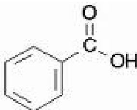
Figura 2 – Estrutura do ácido benzóico
