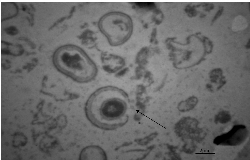
Figura 12 – Visualização da degradação total da célula de Alicyclobacillus acidoterrestris tratados com ácido benzóico (0,5g/mL) por Microscopia Eletrônica de Transmissão, após 4horas, à 45°C, indicada por setas.
