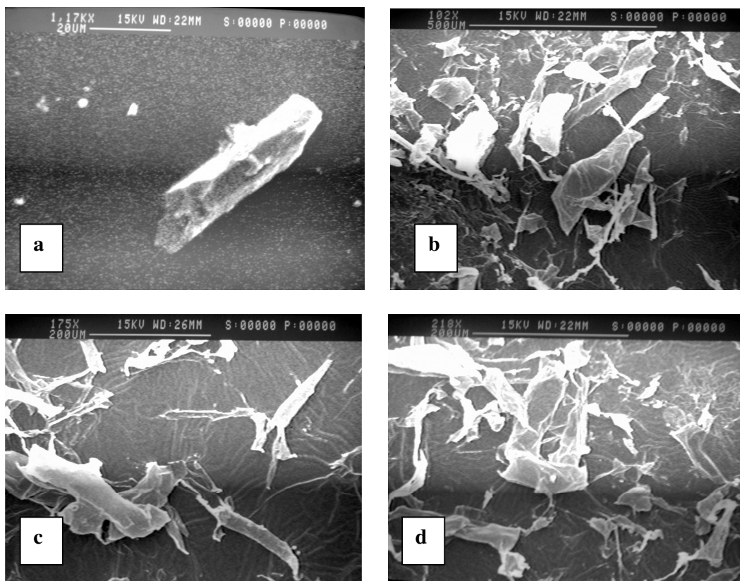
Figura 6 - Fotomicrografias obtidas por MEV do ácido benzóico micronizado. a) cristal de ácido benzóico isolado com diâmetro de ca 10µm, visualização feita em 1,17 k e 15kv por MEV. b ) cristais alongados com distribuição irregular de tamanho (102x e 15kv). c) cristais alongados com distribuição irregular de tamanho (218x e 15kv). d ) cristais alongados com distribuição irregular de tamanho (175x e 15kv).
