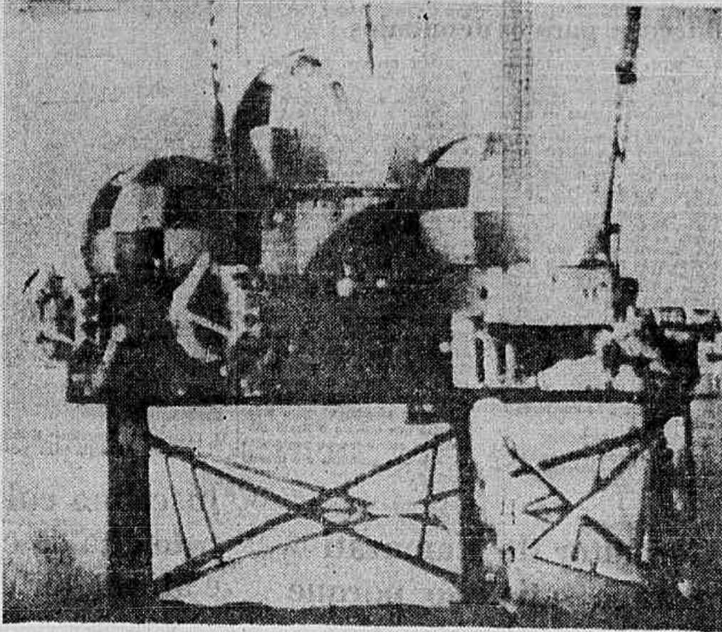
A torre de radar flutuante da Força Aérea dos Estados Unidos, que naufragou ao largo de Nova Jersey com 28 homens em seu interior. (Radiofoto da AP, especial para o JORNAL DO BRASIL)
