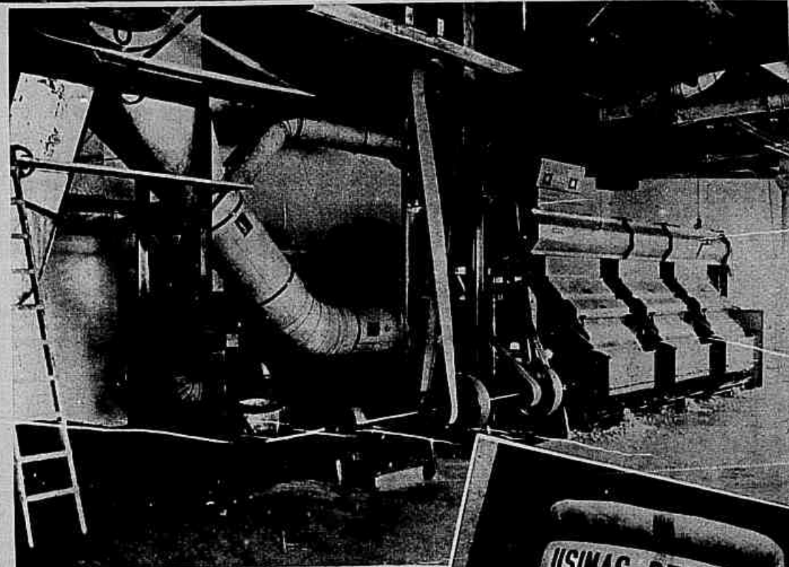
Um dos grupos de descaroadores, inteiramente pneumático, typo "Hardwick" com capacidade para descaroador tres mil kilos por hora, ou sejam 10 mil kilos de pluma por dia.
