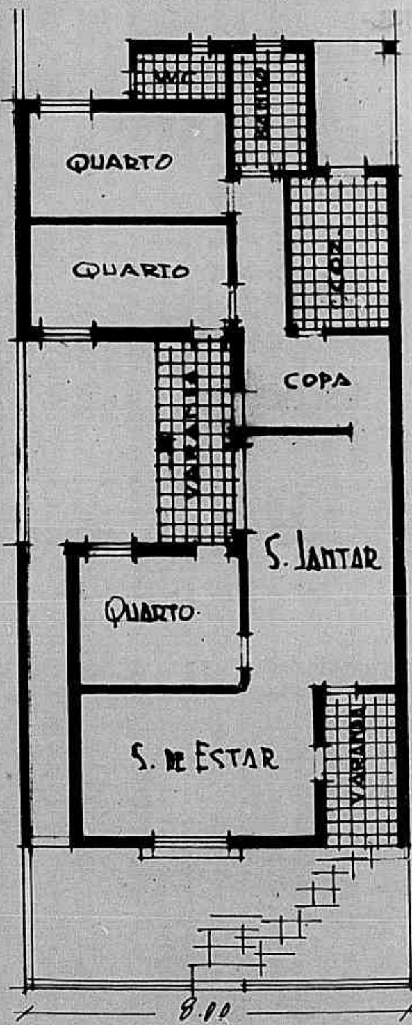
Projecto de construção rustica sobre um terreno de oito metros de frente.
