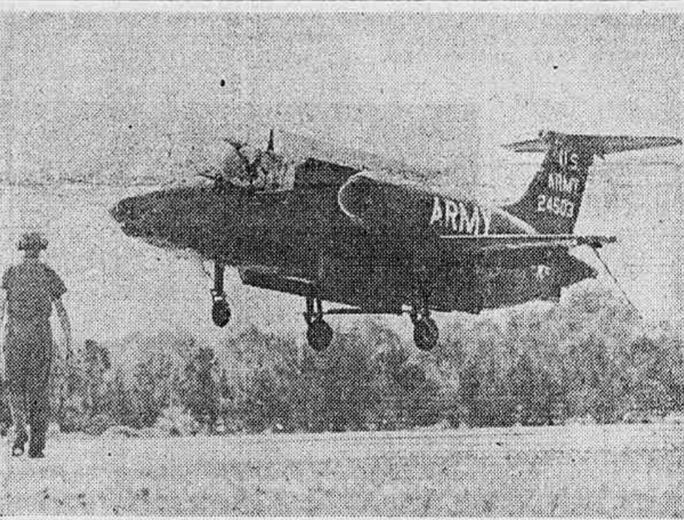
«BEIJA-FLORES» É AVIÃO E HELICÓPTERO — Este avião, que está sendo submetido a provas pelo Exército dos Estados Unidos, é o XV-4A «Hemmingbird» (Beija-Flor), capaz de levantar vôo como um helicóptero e desenvolver uma velocidade de 800 quilômetros por hora. O XV-4A é movido a jato e fabricado pela «Lockheed».
