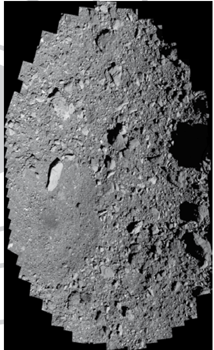
Az OSIRIS-Rex másodlagos mintavételi célpontterületéről készült rendkívül részletes felvétel (NASA)
