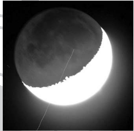
2020.03.29. 20:34 – Starlink áthúzás a Hold előtt. Akkor szél volt, hogy nem nagyon tudtam fotózni (10–15 képenként lett egy „használható”), épp be akartam pakolni, amikor megláttam, hogy jön a Starlink konvoj. Egy át is húzott a Hold előtt, amit sikerült elkapni. A szél miatt nagyon életlen a kép. SW 90/900, EQ2, Nikon D3200, ISO 200, 5 s (Molnár Attila felvétele Budapestről készült)
