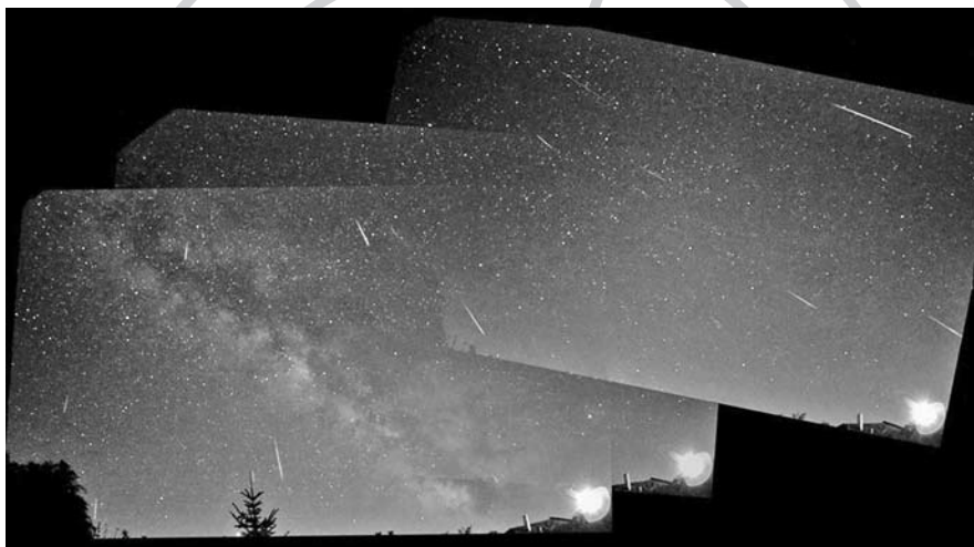
Lyrida meteorok az április 22/23-i éjjelen, Gucsik Bence mozaikfelvételén
