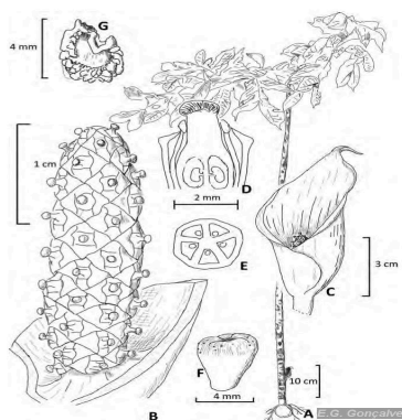
Figura 1: Dracontium narae E.G.Gonç.
