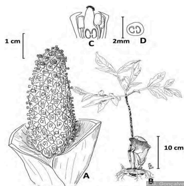
Figura 1: Dracontium laetum E.G.Gonç. & S.P.Santos
