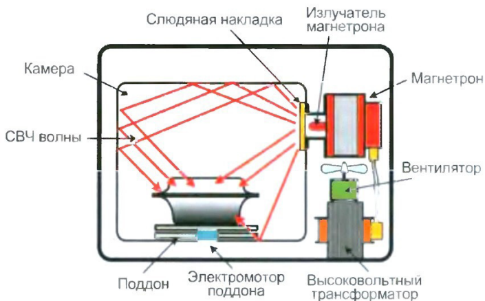
Рис. 1 Устройство СВЧ-печи
