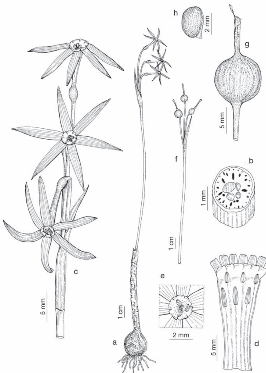
Lám. 74.— Narcissus viridiflorus , a, c, e) La Línea de la Concepción, Cádiz (MGC 52828); b, d) San Roque, Cádiz (MA 777850); f-h) Los Barrios, Cádiz (SEV 124371): a) hábito; b) sección transversal del escapo; c) inflorescencia y espata; d) tubo de la corola abierto, con los 2 verticilos de estambres; e) corona, vista cenital; f) infrutescencia; g) cápsula; h) semilla.
