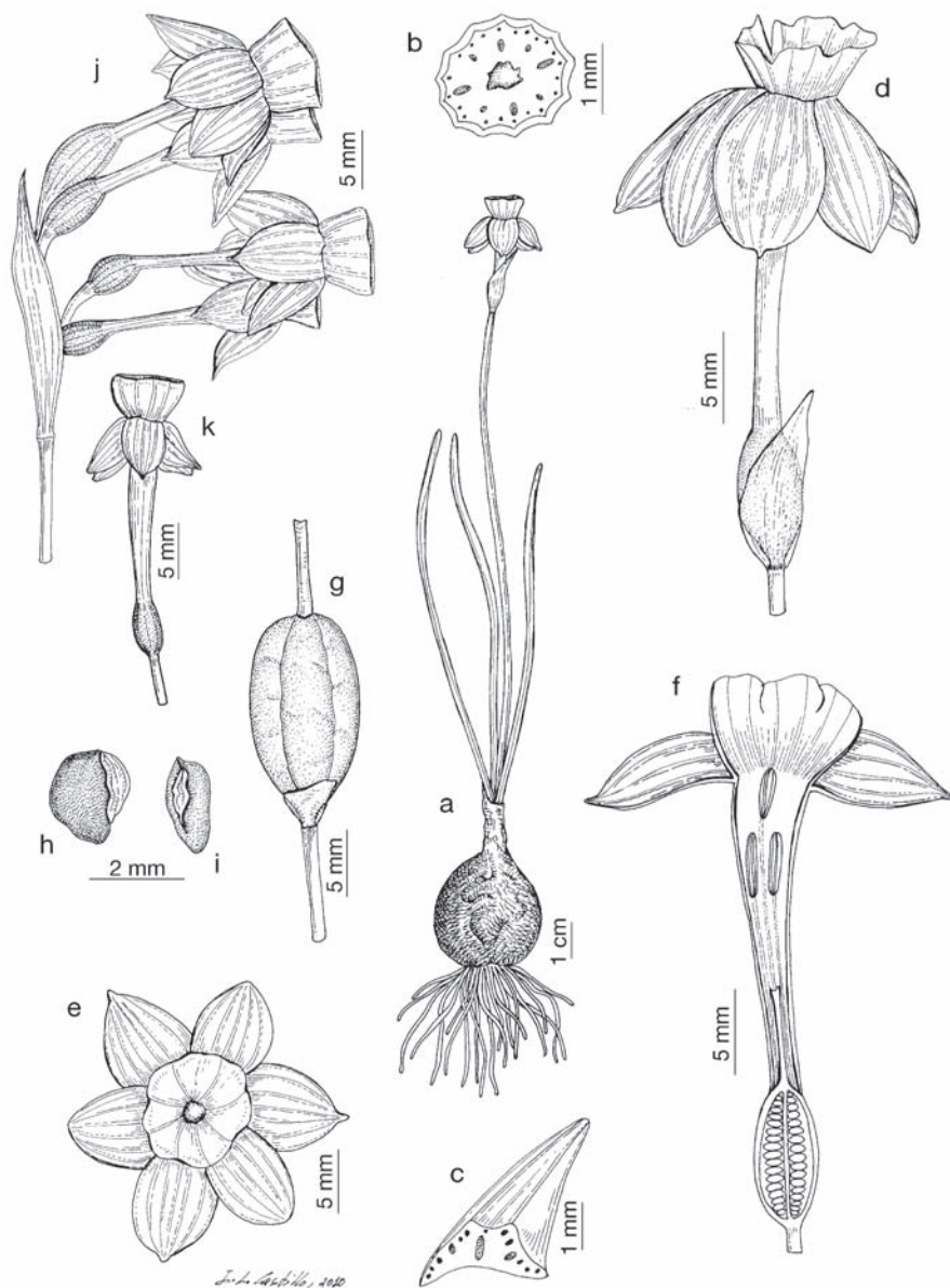
Lám. 78.— Narcissus rupicola , a, g-i) Casillas, Ávila (MA 588140); b-f) San Rafael, Segovia (MA 764860): a) hábito; b) sección transversal del escapo; c) fragmento de una hoja con detalle de su sección transversal; d) flor y espata, vista lateral; e) flor, vista cenital; f) sección longitudinal de una flor; g) cápsula; h, i) semillas. N. scaberulus subsp. calcicola , Minde, Ribatejo (MA 784464): j) inflorescencia y espata. N. scaberulus subsp. scaberulus , Oliveira do Conde, Beira Alta (MA 784548): k) flor, vista lateral.
