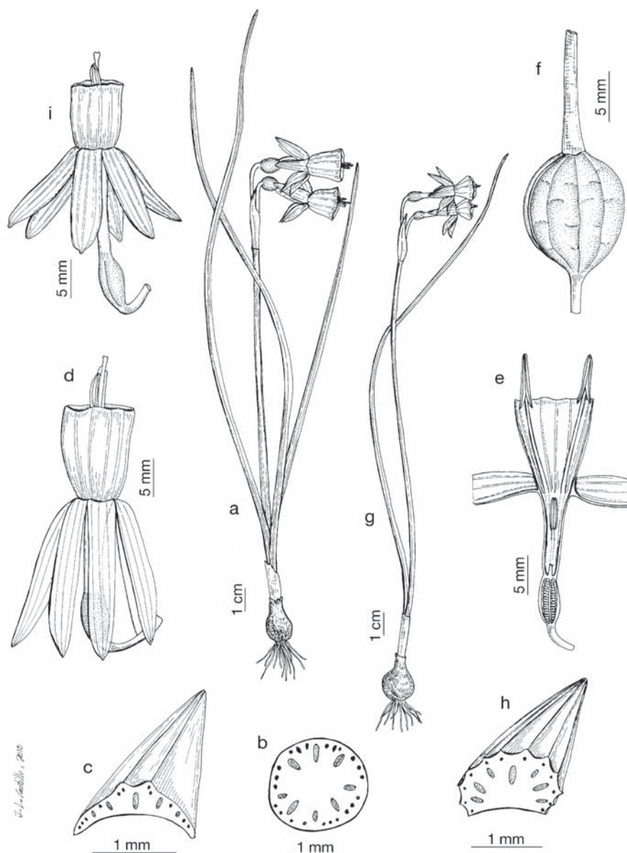
Lám. 79.— Narcissus triandrus subsp. triandrus , a, d-f) Carnota, La Coruña (MA 565168); b, c) Senhora da Peneda, Minho (MA 768567); a) hábito; b) sección transversal del escapo; c) fragmento de una hoja con detalle de su sección transversal; d) flor, vista lateral; e) sección longitudinal de una flor; f) cápsula. N. triandrus subsp. pallidulus , g) Montánchez, Cáceres (MA 728422); h, i) El Escorial, Madrid (MA 764863); g) hábito; h) fragmento de una hoja con detalle de su sección transversal; i) flor, vista lateral.
