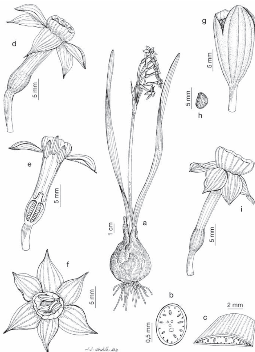
Lám. 75.— Narcissus pachybolus , a-c) Sorbas, Almería (MA 226135); d-f) Mazarrón, Murcia (MA 784724); g, h) Sorbas, Almería (MA 208486): a) hábito; b) sección transversal del escapo; c) fragmento de una hoja con detalle de su sección transversal; d) flor en vista lateral; e) sección longitudinal de una flor; f) flor, vista cenital; g) cápsula; h) semilla. N. dubius , Sax, Alicante (MA 784450): i) flor, vista lateral.
