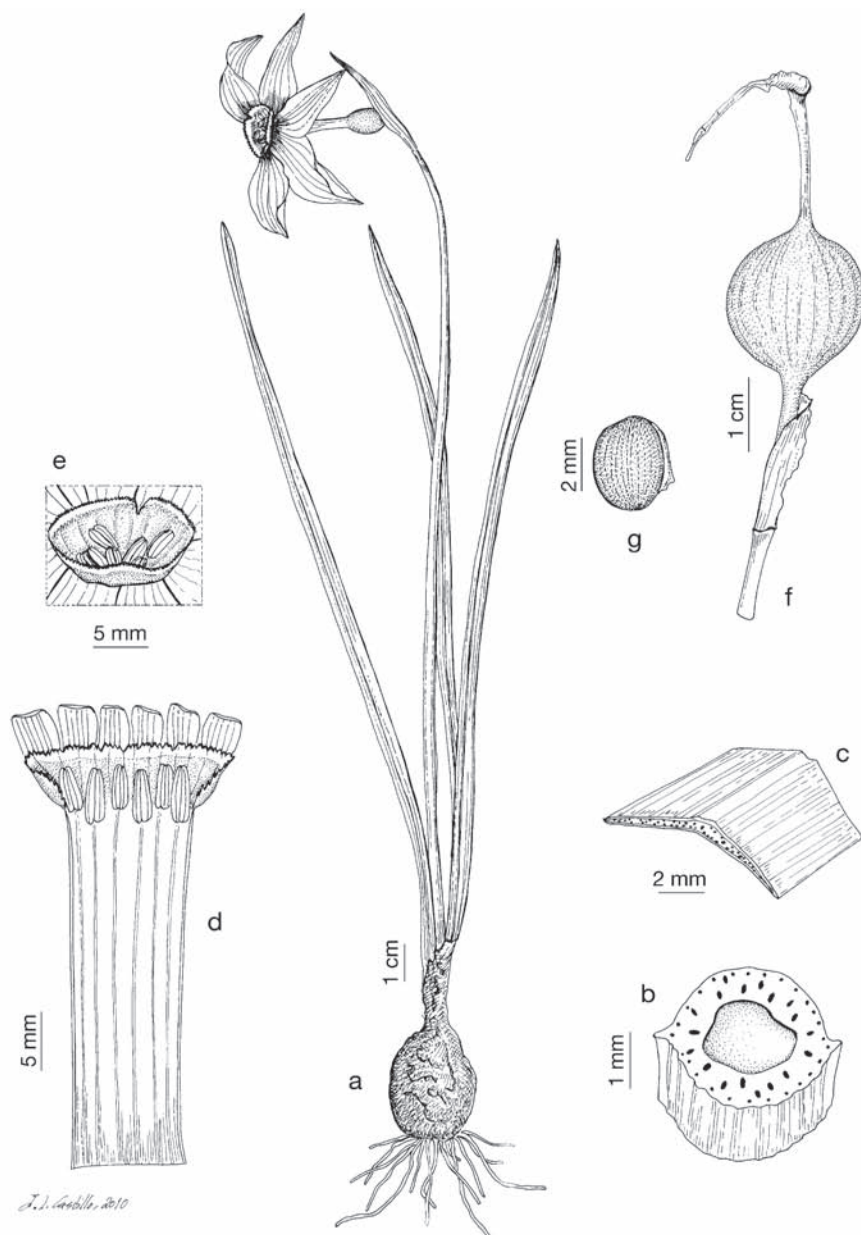
Lám. 76.— Narcissus poeticus , a, c, d) Vall d'Incles, Andorra (MA 755653); b, e) Ordino, Andorra (MA 755654); f, g) Espot, Lérida (BCN 47857): a) hábito; b) sección transversal del escapo; c) fragmento de una hoja con detalle de su sección transversal; d) tubo de la corola abierto, con los dos verticilos de estambres; e) corona; f) cápsula y espata; g) semilla.
