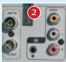
Die Unterschiede liegen im Detail: Die Signale des zweiten Tuners werden über einen zusätzlichen Cinch-AV-Ausgang bereitgestellt – wahlweise steht am UHF-Antennenausgang Tuner 1 oder 2 bereit.
