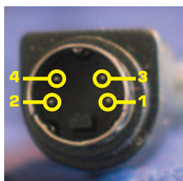
Hosiden-Stecker für S-Video (Y/C)-Verbindung (s. unten)
