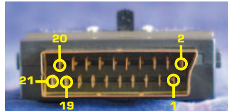
SCART-Stecker: Übertragung nach FBAS, Y/C oder RGB-Norm (s. links)
