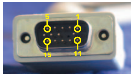
Die vom PC her bekannten VGA-Stecker mit 15 Polen ermöglichen beste Bild- qualität (s. links unten)
