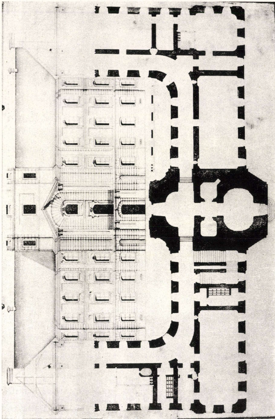
1. ábra. Gerl alap- és homlokrajza, az 1765-ben építeni kezdett toronyrészről, annak udvari homlokzatáról, Gerl kisebb ajtó- és ablakméreteivel.
