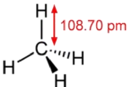
Molécula de metano
