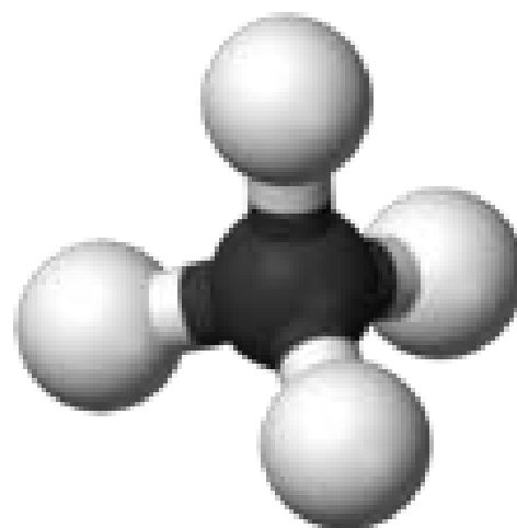
Molécula de metano
