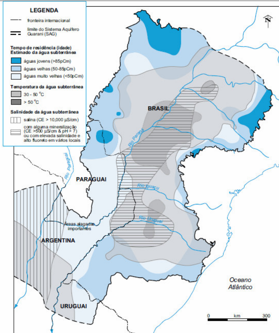
Figura 3.2/43: Variações da temperatura e da salinidade das águas do Sistema Aquífero Guarani, e idade das águas subterrâneas, datada por \delta^{14}C (porcentagem de carbono moderno - pCm). Fonte: Foster et al. (2009).
