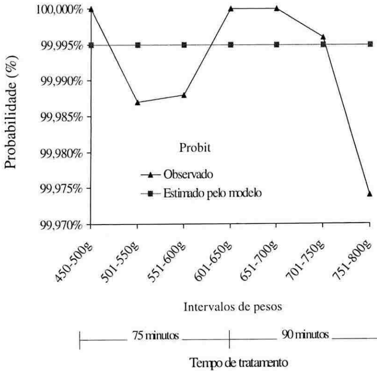
Figura 1. Resultado da análise de Probit, para frutos com pesos variando de 450-800g, infestados por larvas de 3 a estágio e tratados em água a 46,1±0,5°C por 75 e 90 minutos.
