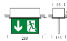
Deckeneinbaumont
