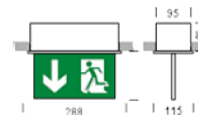
Deckeneinbaumont
