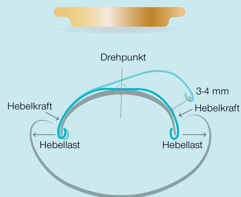
VOLLSPANGE
