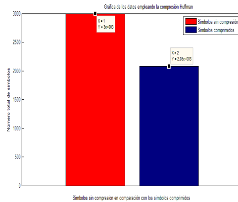
Fig. 4 Resultado de una compresión de datos Huffman
