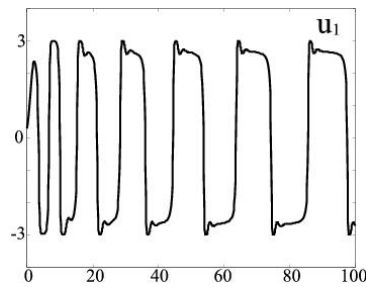
Fig. 16. Destabilizing input
