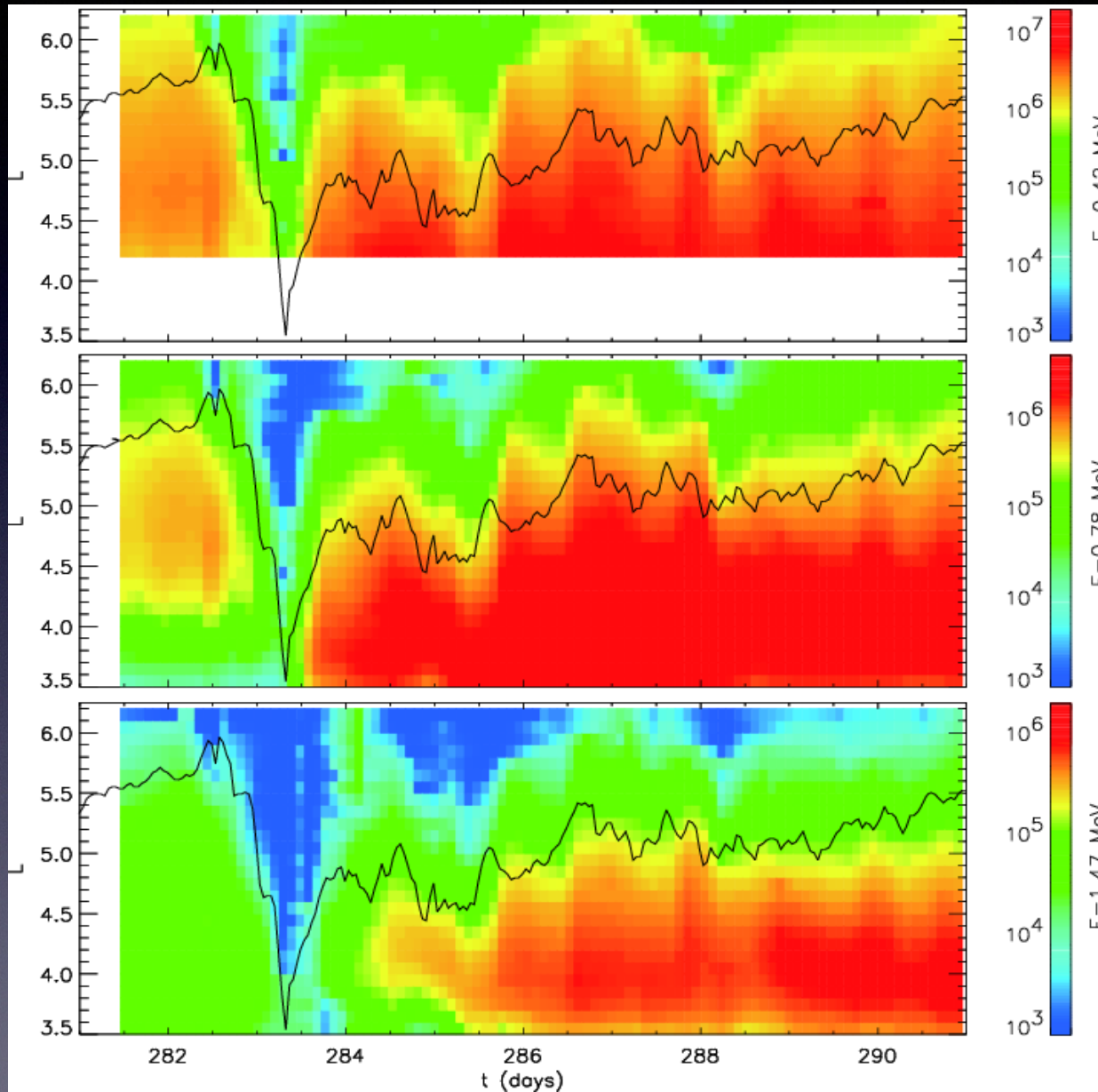
1990年10月8日磁暴期间CRRES卫星观测结果 [Albert et al., 2009]
