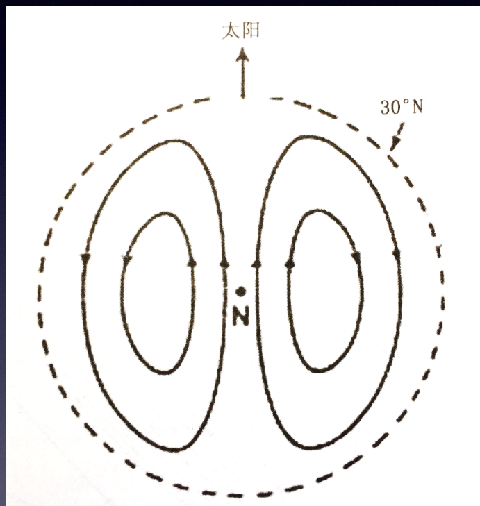
S_q^p 电流系的基本形式
