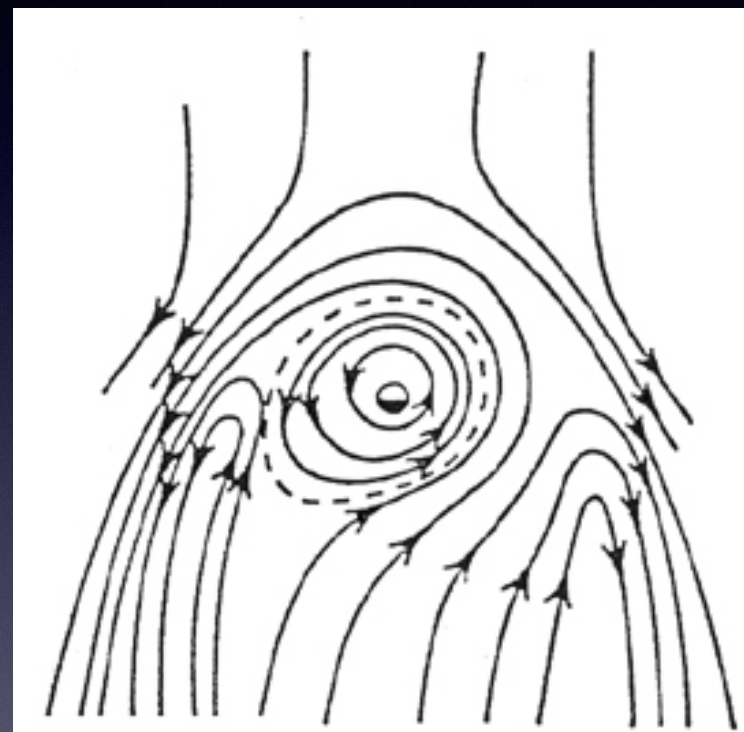
考虑自转的赤道平面磁层环流
