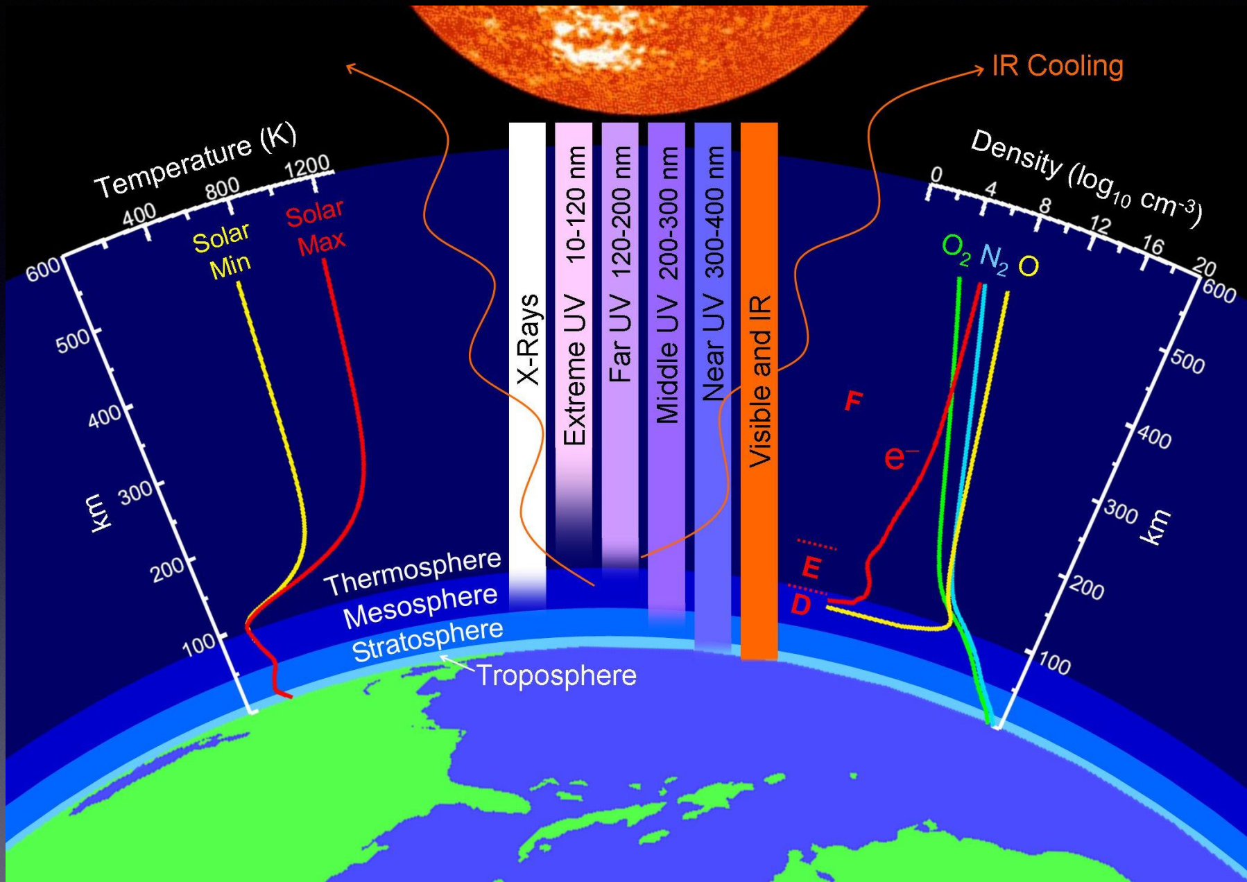
大气温度随高度的变化
