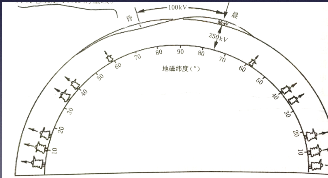
全球大气电路的球形电容器模型
