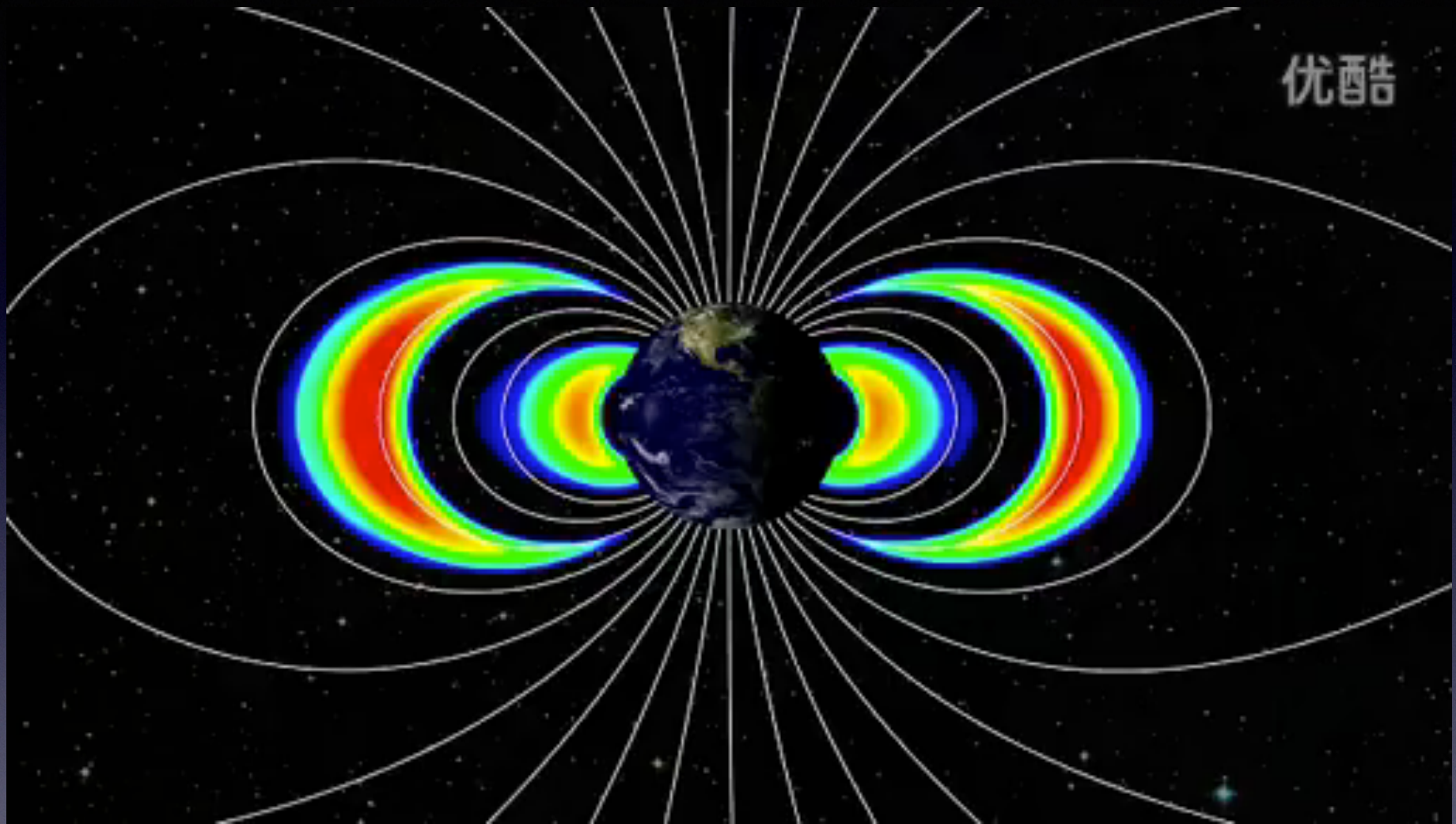
Van Allen卫星探测到的地球辐射带变化
