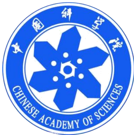
基础研究
