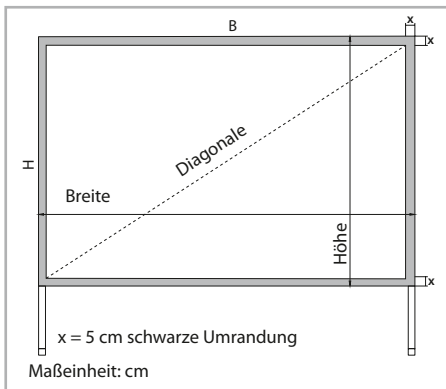
Leinwandfolie mit 5 cm breiter, schwarzer Randverstärkung
