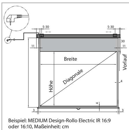
MEDIUM Design-Rollo Electric IR, Infrarotsteuerung mit Handsender und Netzstecker oder Wandbedienteil
