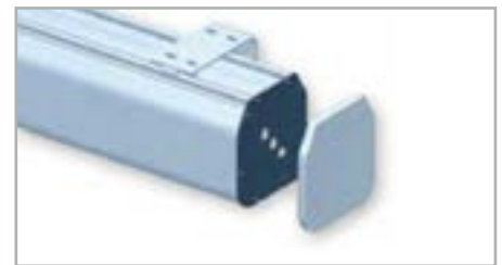
Kompaktes, leichtes Aluminium-Gehäuse mit verschiebbaren Montagewinkeln
