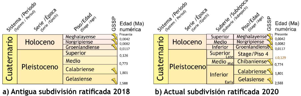
Figura 1. Intervalo del Cuaternario en la tabla cronoestratigráfica Internacional del ICS mostrando: a) la subdivisión estratigráfica hasta mayo de 2019, y b) el esquema actualmente ratificado. La edad anterior para la base del Pleistoceno medio (0,773 Ma) se basa en la del límite Matuyama-Brunhes mientras que su edad actual (0,774 Ma) es la del GSSP de Chiba que se produce antes, 1,1 m por debajo de este límite. La edad provisional actual para la base del Pleistoceno superior (ca. 0,129 Ma) refleja un fuerte aumento de las temperaturas justo antes del máximo calentamiento durante el Último Interglacial (Head, 2019) aunque no está ratificado. Consultar tabla 2 para el código de colores. Traducido y Modificado de Head et al. (2021).
