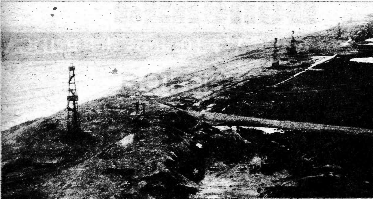
Nuevos pozos de petróleo en Odoptu, isla de Sajalín, perforados en la costa del mar de Ojotsk.
