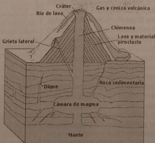
Un volcán sería como un edificio constituido de materiales de origen ígneo acumulados.
