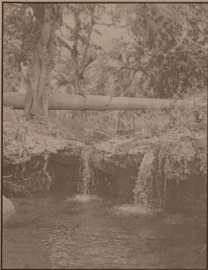
Para que el agua siga corriendo y frenar el impacto de sequías como la pasada, habrá que continuar la reforestación.
