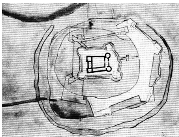
Nicolo Angelini felmérése és bővítési tervrajza a várdai várról 1569-70.
