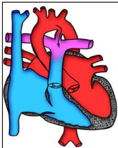
PCA
