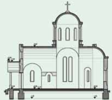
ПОДУЖНИ ПРЕСЕК
