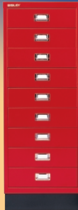
9 Schubladen H 83 mm ohne Schloss, auf Sockel 940 x 349 x 483 mm BA 3/9NL-
