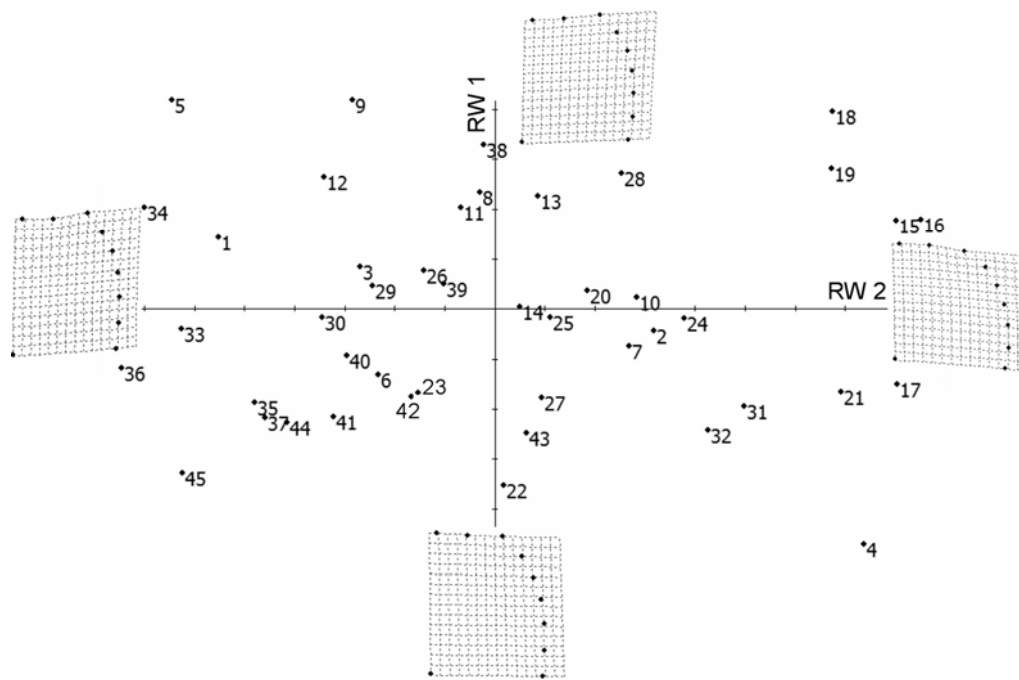
a) Pronotum
