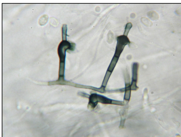
Obr. 4. Zygosporium mycophilum - konidiofor s konidiogenními buňkami a hyalinními konidii (zvětšení 12,5 x 40)
