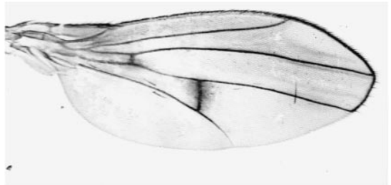
laevacerca
