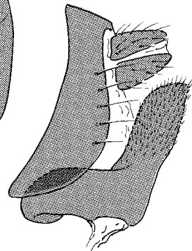
uniradiata
