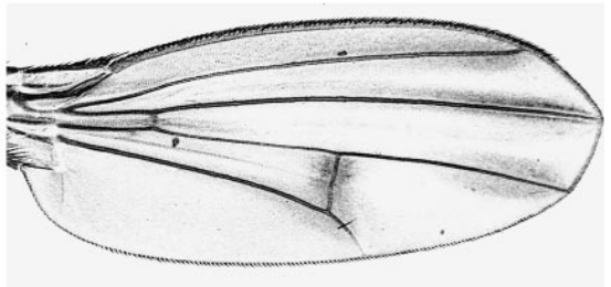
venebula
