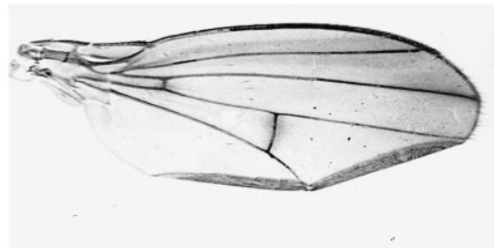
ostia
