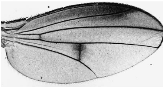
spira
