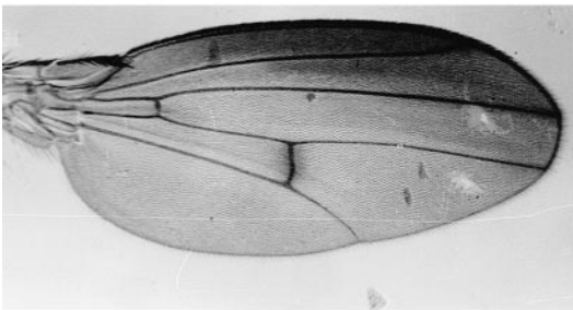
inversa
