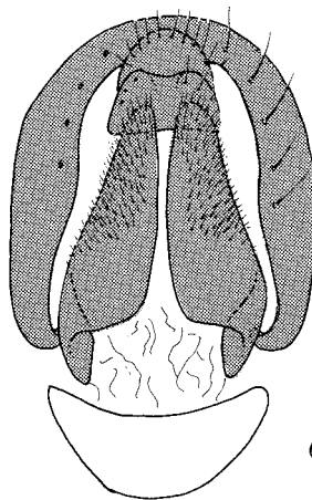
uniradiata
