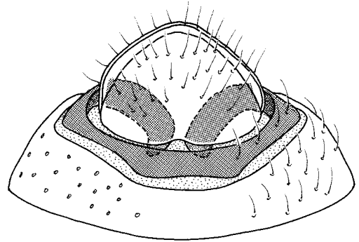
neoinversa
