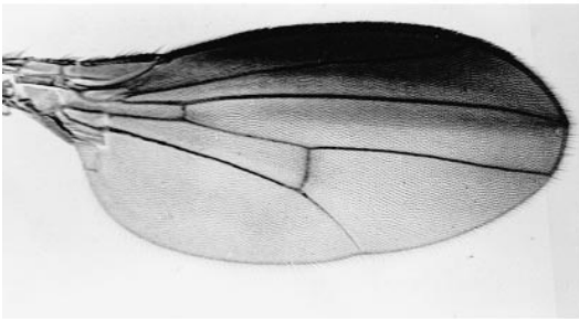
florinversa
