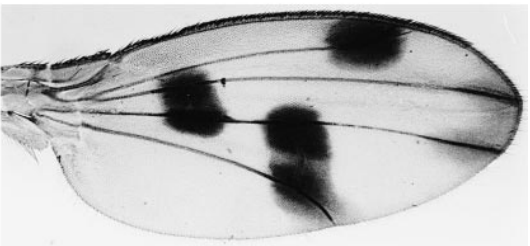
abarista
