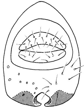
paulhansonii
