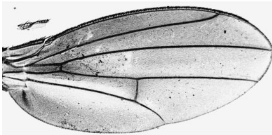
uniradiata
