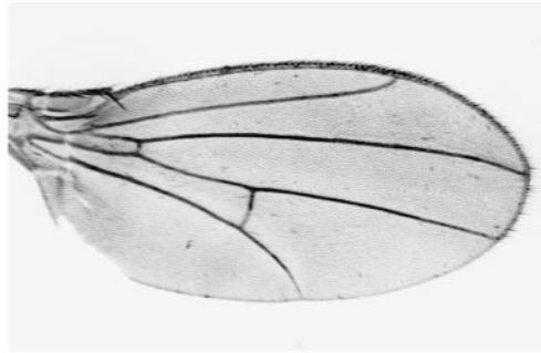
diminuta
