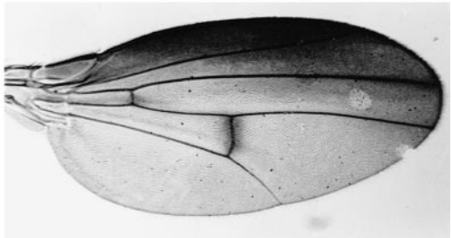
sturtevantii
