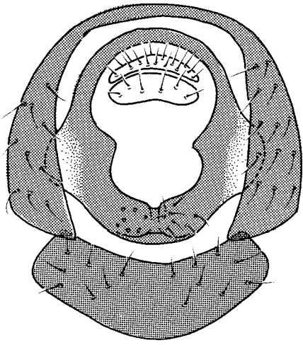
obunca
