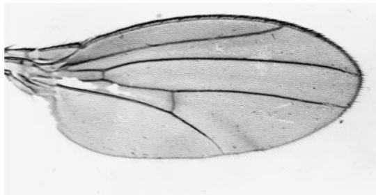
vivipara
