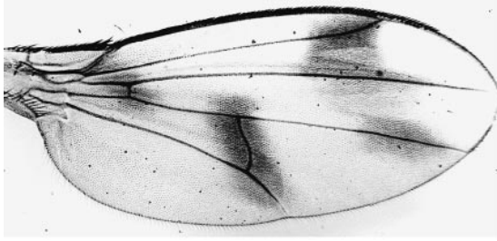
bomplandi
