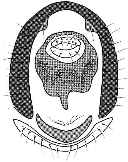
pseudunca
