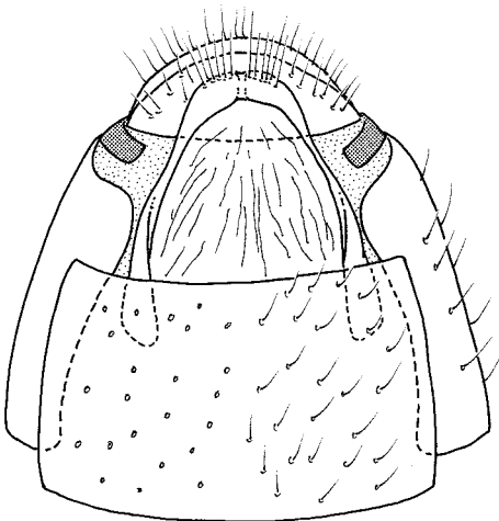
paradoxa
