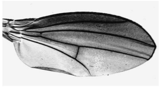
adusta
