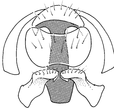
paradoxa
