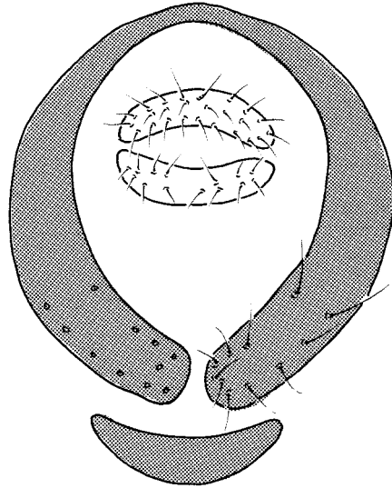
glapica
