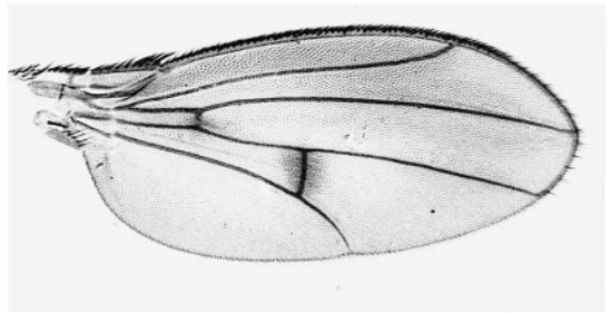
chaeta
