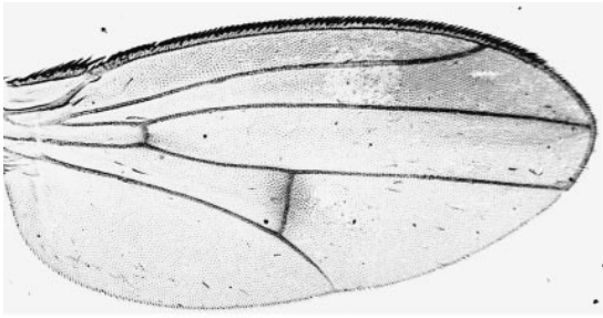
bupeo
