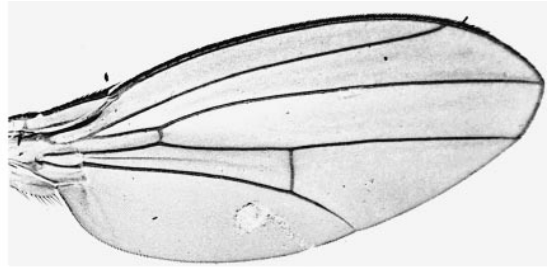
robusta
