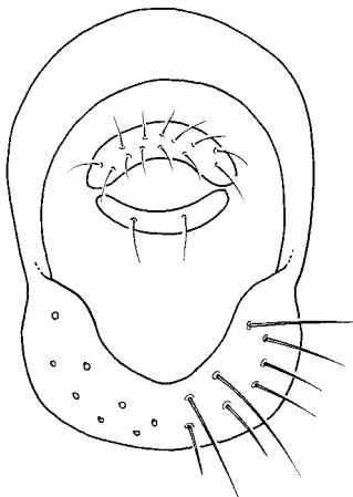
sternospina
