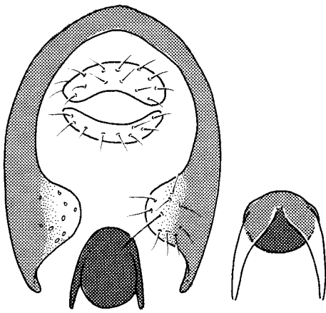
abarista
