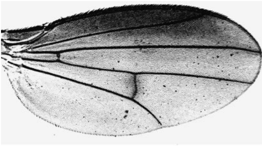
austrinversa
