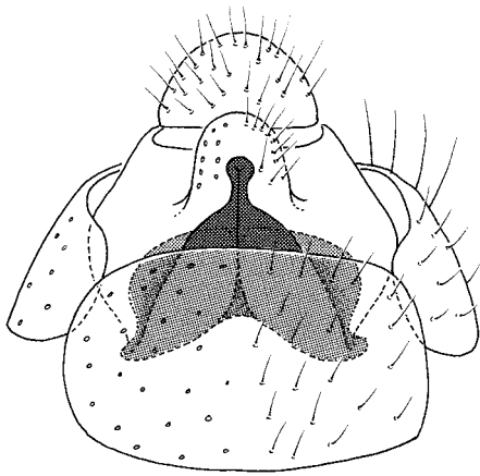
sororia
