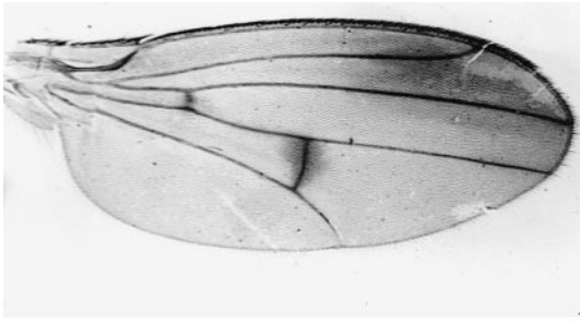
masneri
