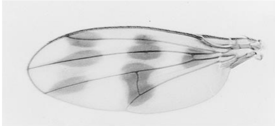
spectabilis
