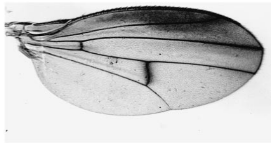
mexinversa
