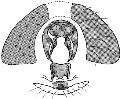
robusta
