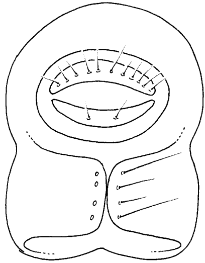
brunnea
