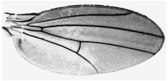
starki
