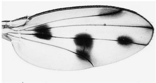
tripunctata
