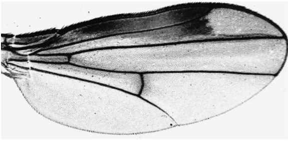
abrupta
