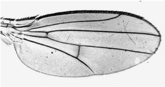
centetor
