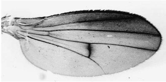
mystaca
