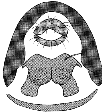
starki
