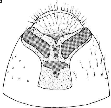
sturtevanti
