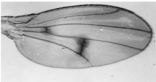
hodita
