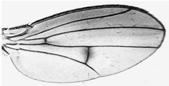
wirthi
