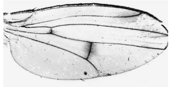
vermes
