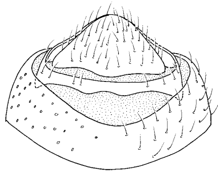
inversa
