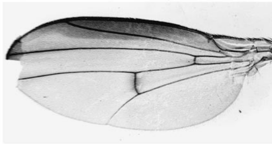
wilhansonii
