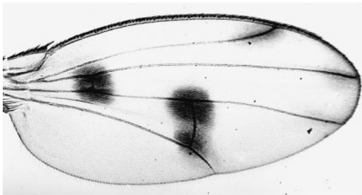
brunnea
