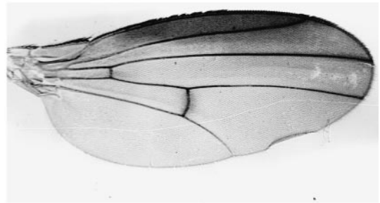
heedi
