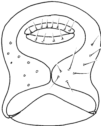
tripunctata
