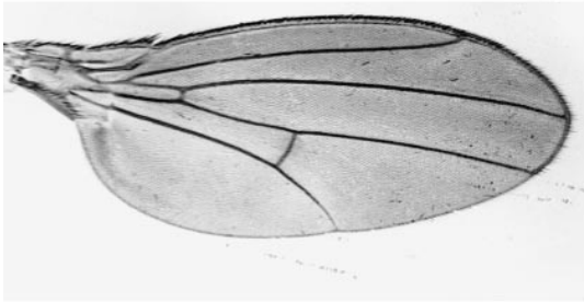
dikra
