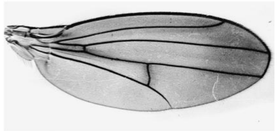
polia
