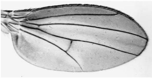
fasciata
