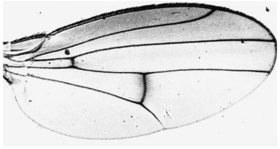
mathisi
