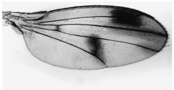
jamaicensis
