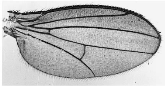
ectopia
