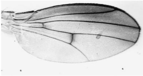
neoinversa
