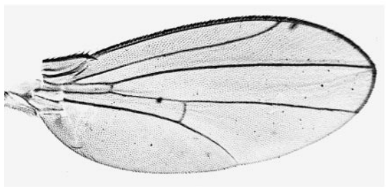
vapida
