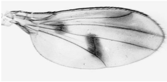
sororia
