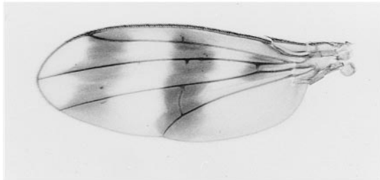
spectabilis
