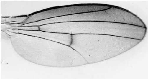
sturtevantii
