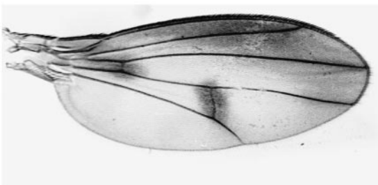
telescopica
