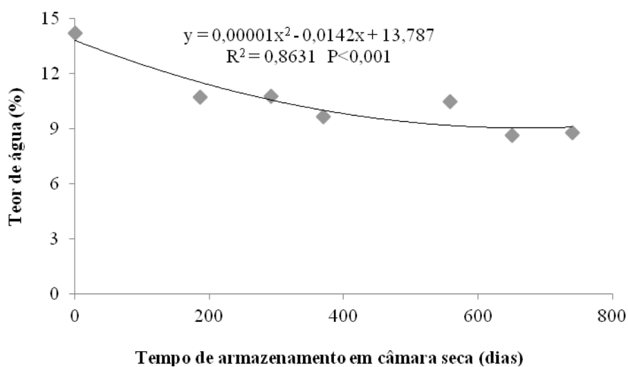
Figura 2. Teor de água de cipselas de S. luzulifolia coletadas em Tapes, RS, durante o período de armazenamento em câmara seca (temperatura constante de 17 °C e umidade relativa do ar de 45 %).
