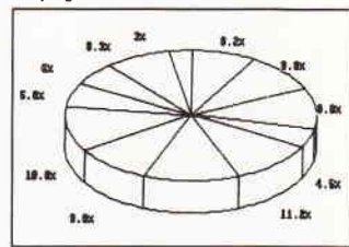
Beispielgrafik STATISTIC-STAR
