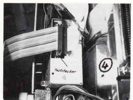
Bild 4: Platzierung des Teststeckers
