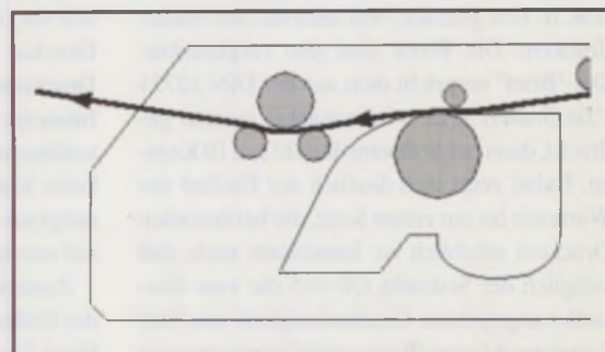
Papierweg beim Seikosha OP-105
