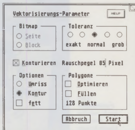
Abb. 1: Die Dialogbox zum Vektorisieren
