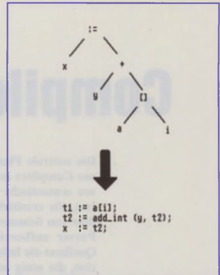
Abb. 1: Strukturbaum und Tupelcode für 'x := y + a[i]'
