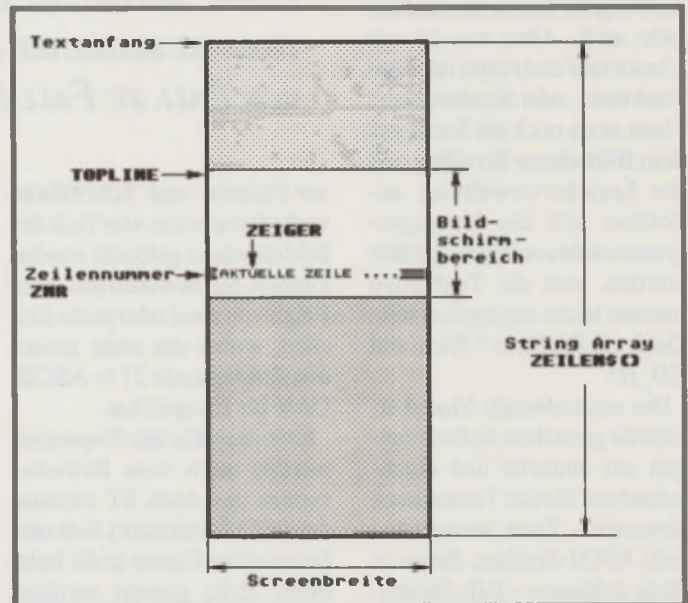
Bild 1: Zusammenhang zwischen Variablen und Textspeicher
