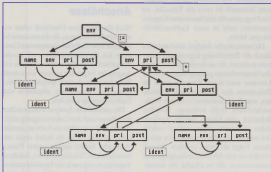
Abb. 3: Abhängigkeiten der Attribute
