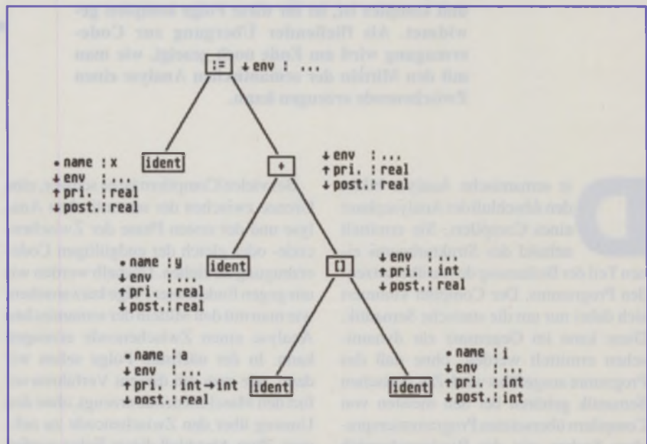
Abb. 2: Attributierter Strukturbaum für 'x := y + a[i]'
